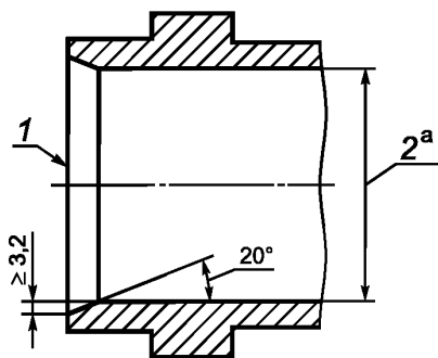
1 — входной торец плунжера; 2 — отверстие втулки; а — допуск номинального
