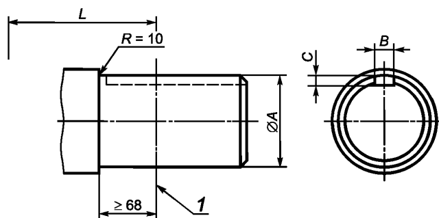
1 — геометрическая ось первого ряда зубьев; А — диаметр вала; В — ширина шпоночного паза; С — глубина шпоночного паза
