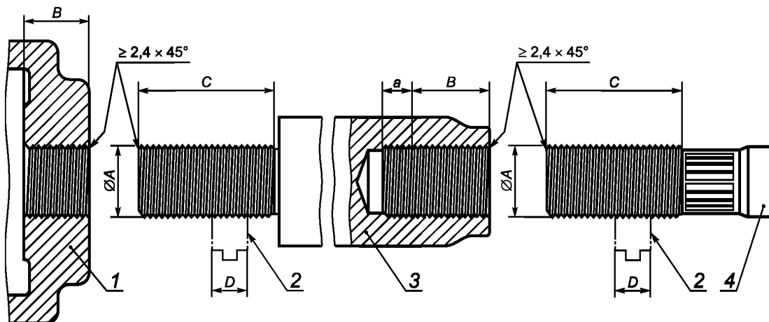
1 — крейцкопф; 2 — контргайка; 3 — удлинение крейцкопфа; 4 — шток плунжера; а — шаг резьбы
