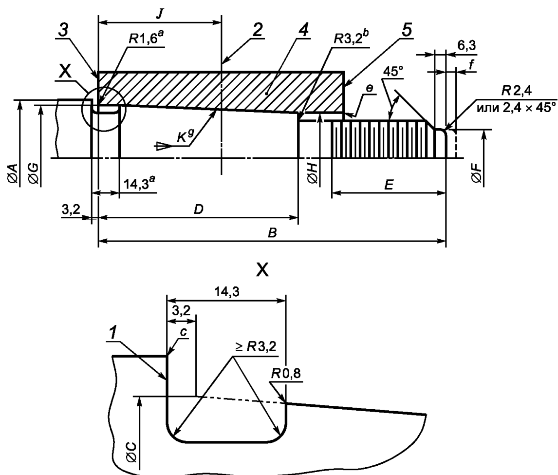
1 — заплечик штока M; 2 — геометрическая ось поршня (в сборе); 3 — заплечик N, заплечик поршня, штоковая полость: a — максимальный размер; b — минимальный размер; c — фаска \leq 0,5 мм; j — длина до центральной оси поршня; B — длина штоковой полости; X — галтель и диаметр выточки, нагартанной при холодной обработке 4 — поршень; 5 — заплечик P, заплечик поршня, конец резьбы: e — фаска; f — максимальное удлинение хвостовика 3,2 мм; g — конус; R — радиус или фаска
