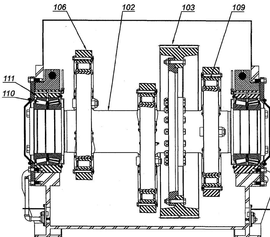
Рисунок В.2 — Поперечное сечение приводной части (номенклатура деталей см. в таблице В.1)
