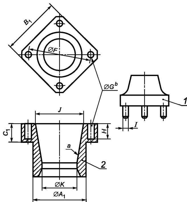
1 — вкладыш ротора под ведущую трубу с ведущими пальцами; 2 — постоянная втулка; a — конусность 1:3 ( 330 \pm 1,5 ) мм/м; b — диаметр поводкового отверстия
