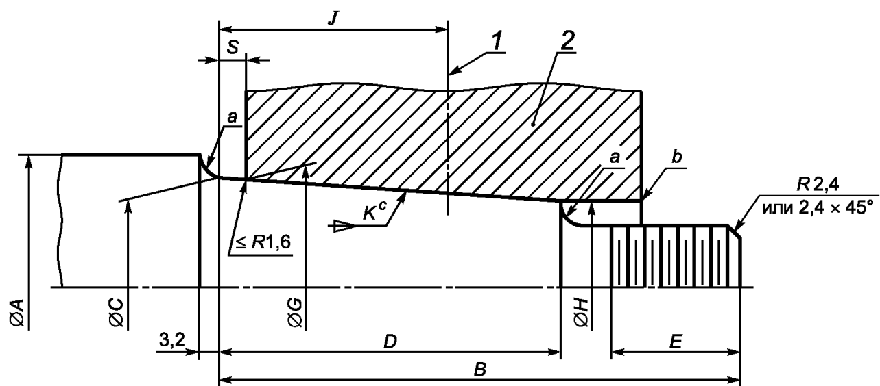
1 — центровая линия поршня (положение после крепления); 2 — поршень; a — галтель, радиус галтели R = 3 мм на каждом выступе поршня; b — фаска; c — конусность
