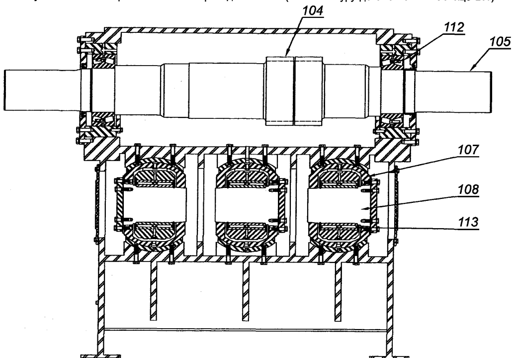
Рисунок В.3 — Поперечное сечение через вал-шестерню и крейцкопф (номенклатура деталей см. в таблице В.1)
