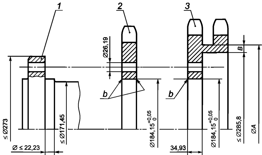
1 — ступица колеса; 2 — одиночное (единичное) колесо; 3 — двойное колесо; a — максимальный диаметр ступицы колеса, обеспечивающий зазор цепной передачи; b — фаска 2 мм · 45°; c — 8 отверстий, равномерно расположенных по диаметру центральной окружности отверстий под болты
