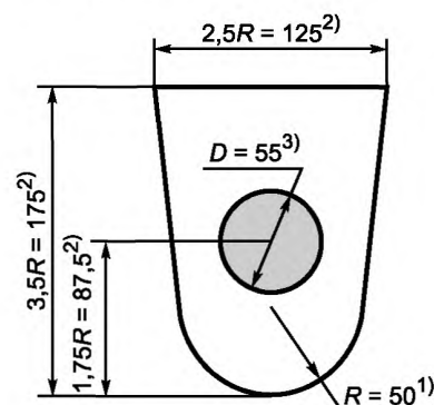
Рисунок 4 — Эквивалентные круговые модели. Сложные формы
