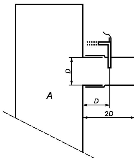
Рисунок 14 — Устройство для отбора проб в приборах типов C_{21} и C_{41}
