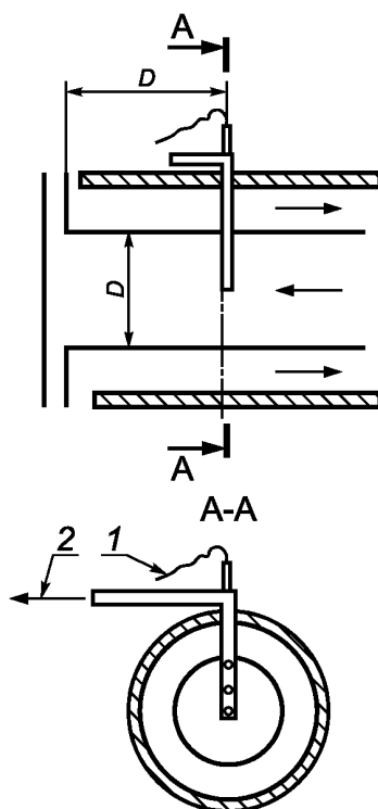
Рисунок 13 — Устройство для отбора проб в приборах типа C_{11}
