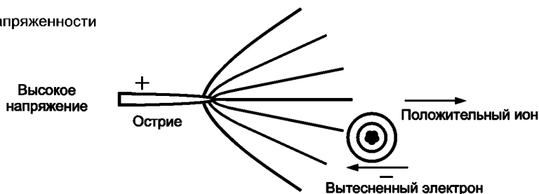
Рисунок 10 — Коронная ионизация — положительная
