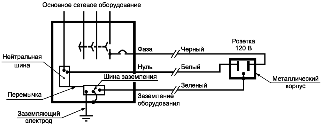
Рисунок 4а — Пример Североамериканской энергосистемы
