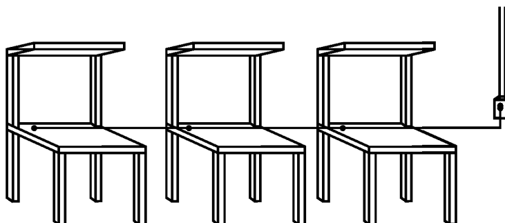
Рисунок 6 — Пример нерекомендуемого заземления последовательно соединенных столов
