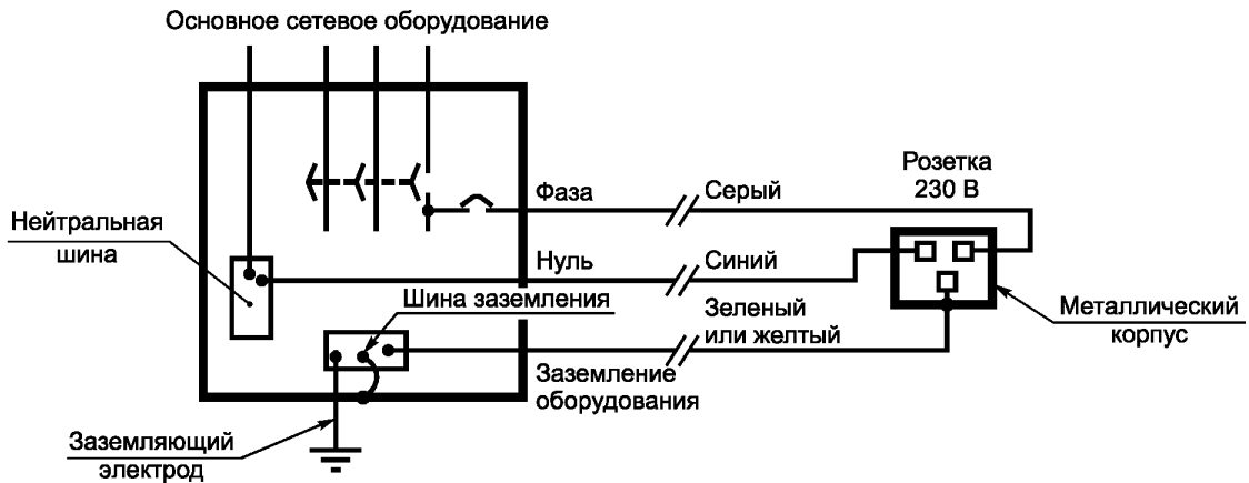
Рисунок 4в — Пример энергосистемы Великобритании — Однофазная система
