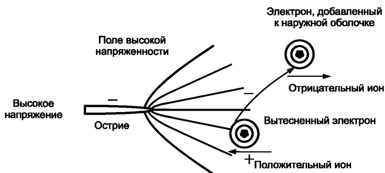
Рисунок 11 — Коронная ионизация — отрицательная
