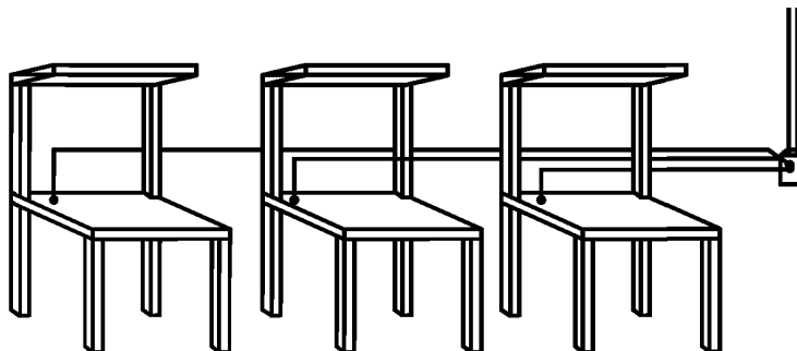
Рисунок 5 — Пример рекомендуемого индивидуального заземления столов
