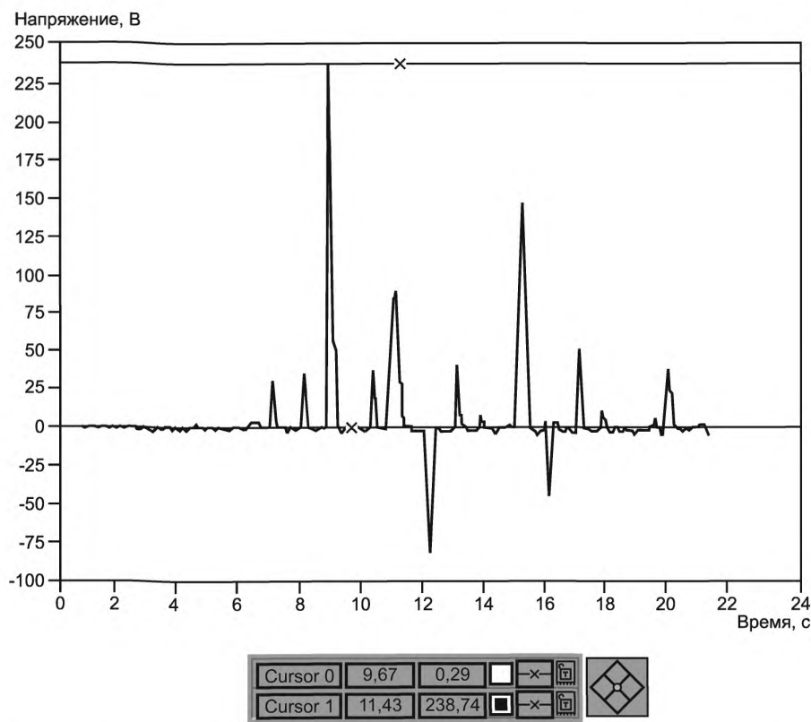
Рисунок 8 — Напряжение на сотруднике, идущем по заземленному проводящему полу с двумя надетыми ремешками заземления
