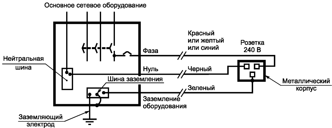
Рисунок 4б — Пример Малазийской энергосистемы
