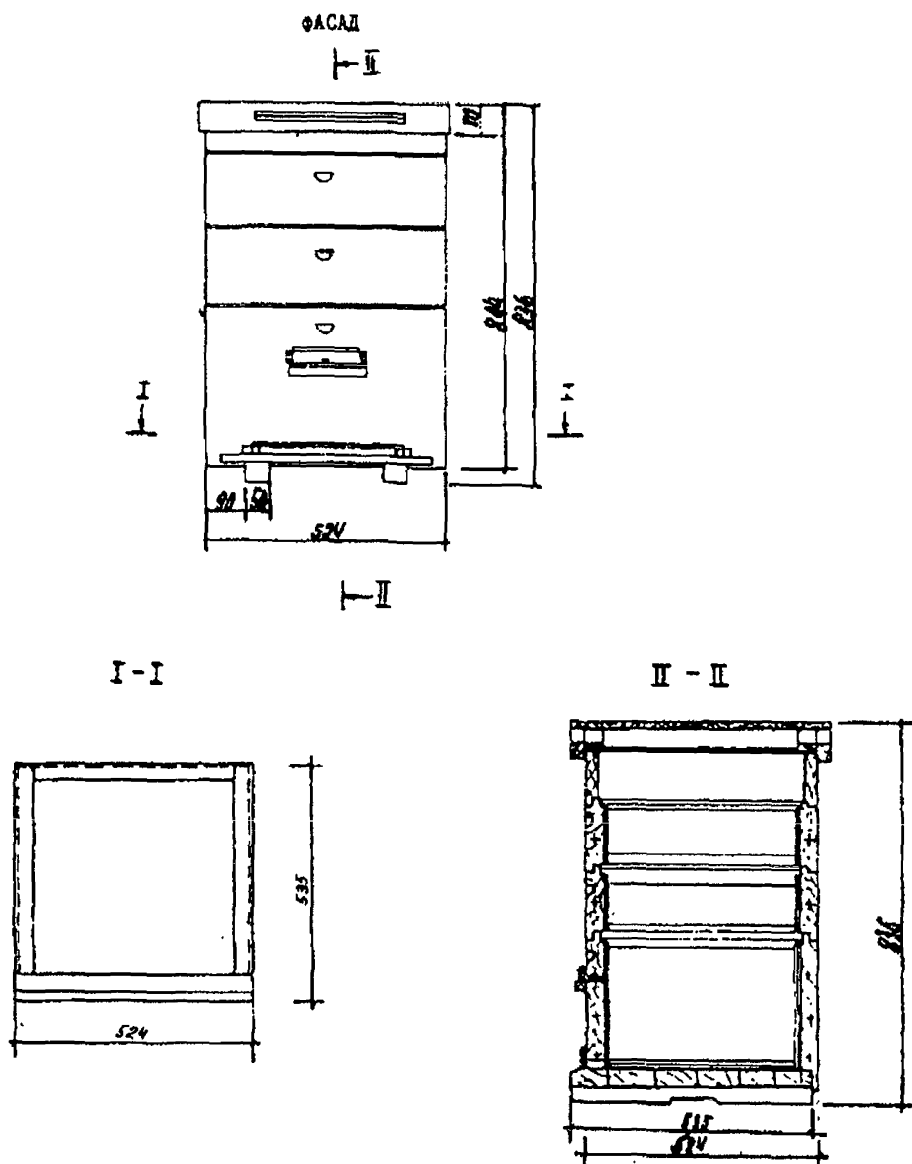
Рис. Е.5. Улей однокорпусный с двумя магазинами (ТП 808-5-14)
