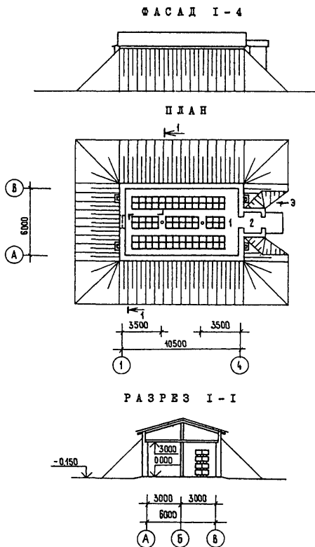
Рис. Д.6. Зимовник на 300 пчелиных семей (ТП 808-5-27.86) наземный: 1-помещение для ульев; 2-тамбур
