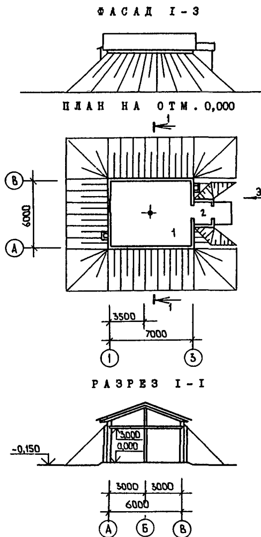
Рис. Д.4. Зимовник на 200 пчелиных семей (ТП 808-5-55.92) наземный: 1-помещение для ульев; 2-тамбур
