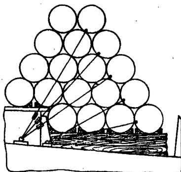
Рис. 2.2.5. Дополнительное крепление бортовых труб
