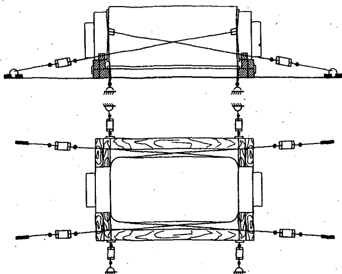
Рис. 2.16.1. Схема крепления вала
