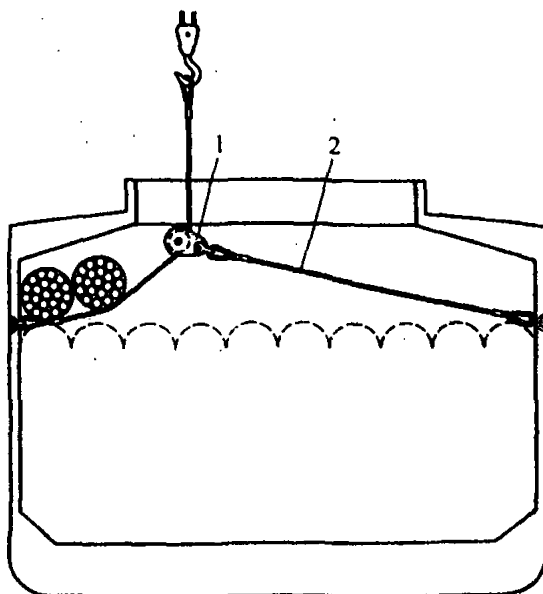
Рис. 2.1.4. Схема применения канифас - блоков при использовании штивирующих стропов:
