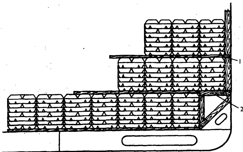
Рис. 2.22.1. Укладка чушек цветных металлов в пакетах:
