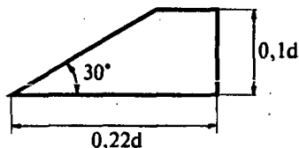
Рис. 2.4.1. Продольное сечение клина: d - наружный диаметр рулона
