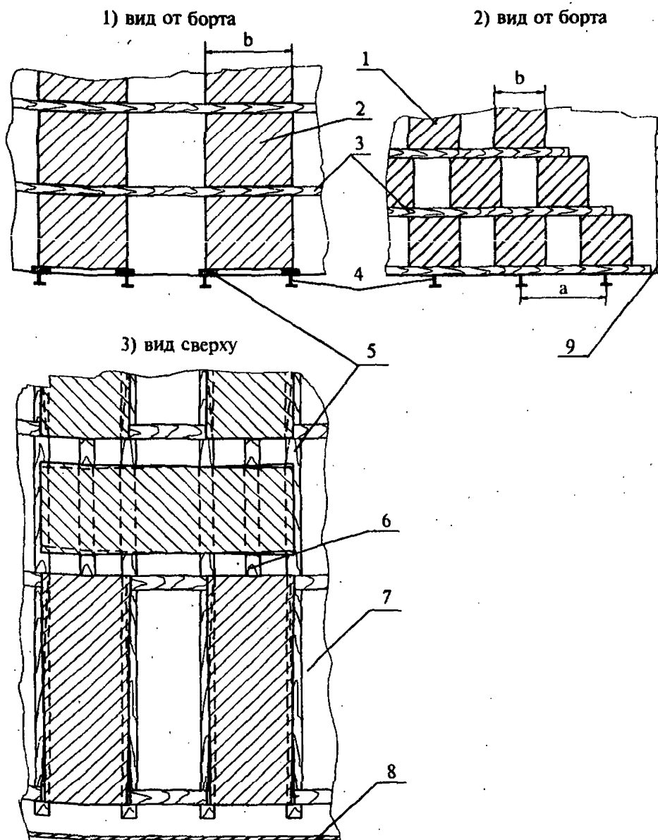
Рис. 2.11.1. Схема размещения:
