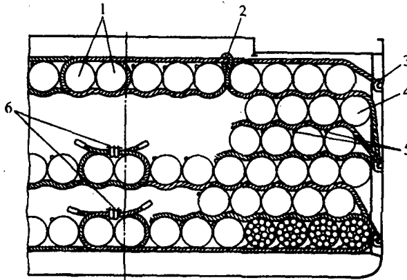
Рис. 2.1.3. Укладка и крепление УГМ с трубами малого диаметра с применением штивиующих стропов:
