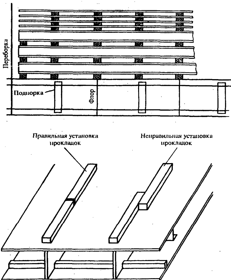
Рис. 2.5.1. Схема установки прокладок на настиле и между листами в штабеле
