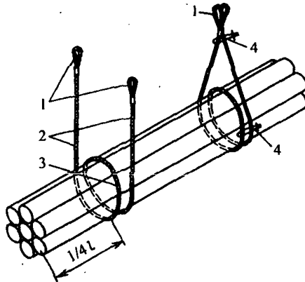
Рис. 2.1.2. Схема формирования УГМ труб малого диаметра в инвентарных стропы способом двойного охвата:
