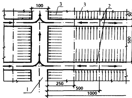
1 – вентилируемый канал; 2 – диффузионные каналы; 3 – движение влаги
