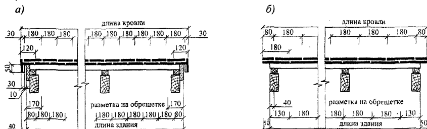
Рисунок К.5 – Продольный разрез кровли с применением на фронте боковой черепицы (а) и без применения такой черепицы (б)
