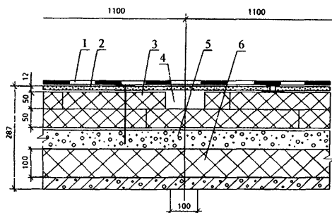
1 – новый кровельный ковер; 2 – сборная стяжка из ЦСП; 3 – минераловатные плиты; 4 – вентилируемые каналы; 5 – существующая стяжка из цементно-песчаного раствора; 6 – увлажненный пенобетон
