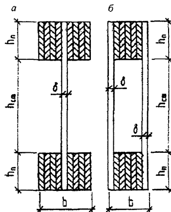
а — двутаврового сечения; б — коробчатого сечения
