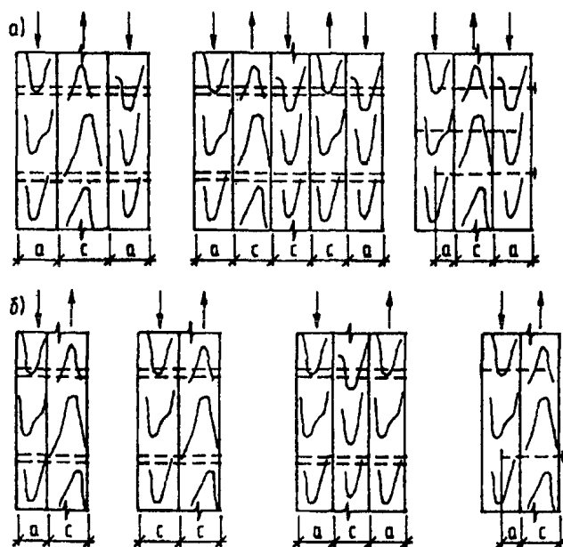
Рисунок 9 — Нагельные соединения
