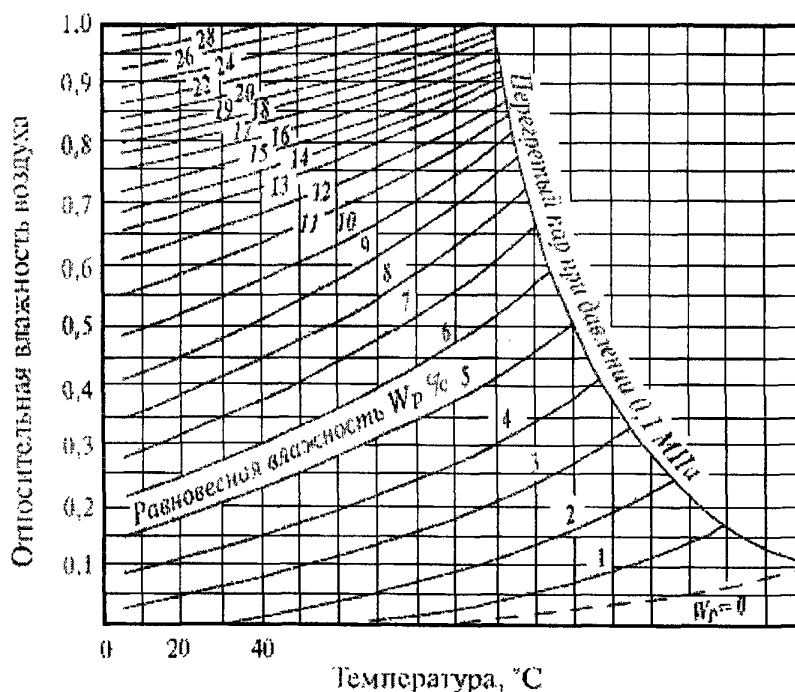
Рисунок Г.1 — Диаграмма равновесной влажности древесины
