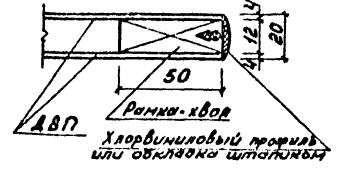
Вариант пустотелого щита.
