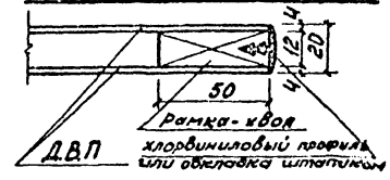
Вариант пустотелого щита
