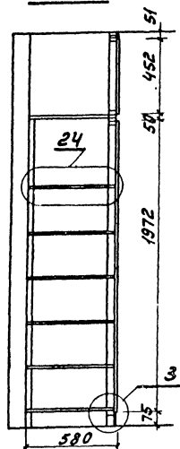
по А-А
