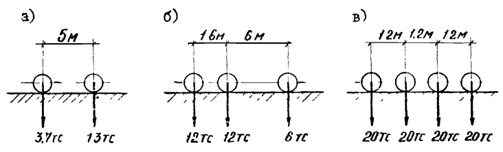
Рис. 7. Схемы временных нагрузок на поверхности грунта для колодцев.
