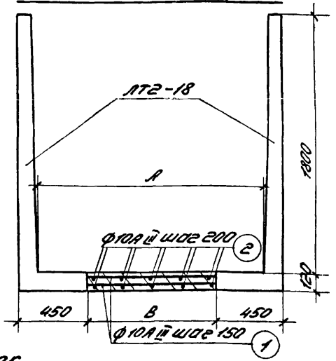
Лоток высотой 1,8м
