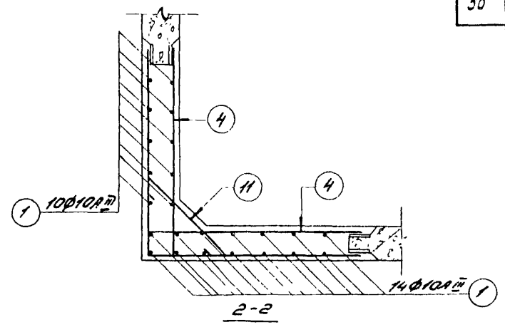
Спецификация арматуры
