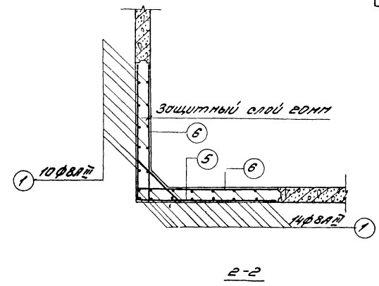
Спецификация арматуры
