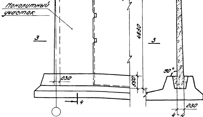
Выборка арматуры на один монолитный участок
