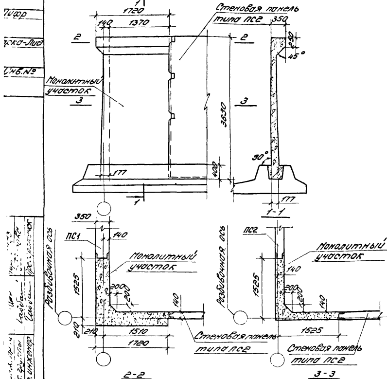
Монолитный участок для стен высотой 3,6 м
