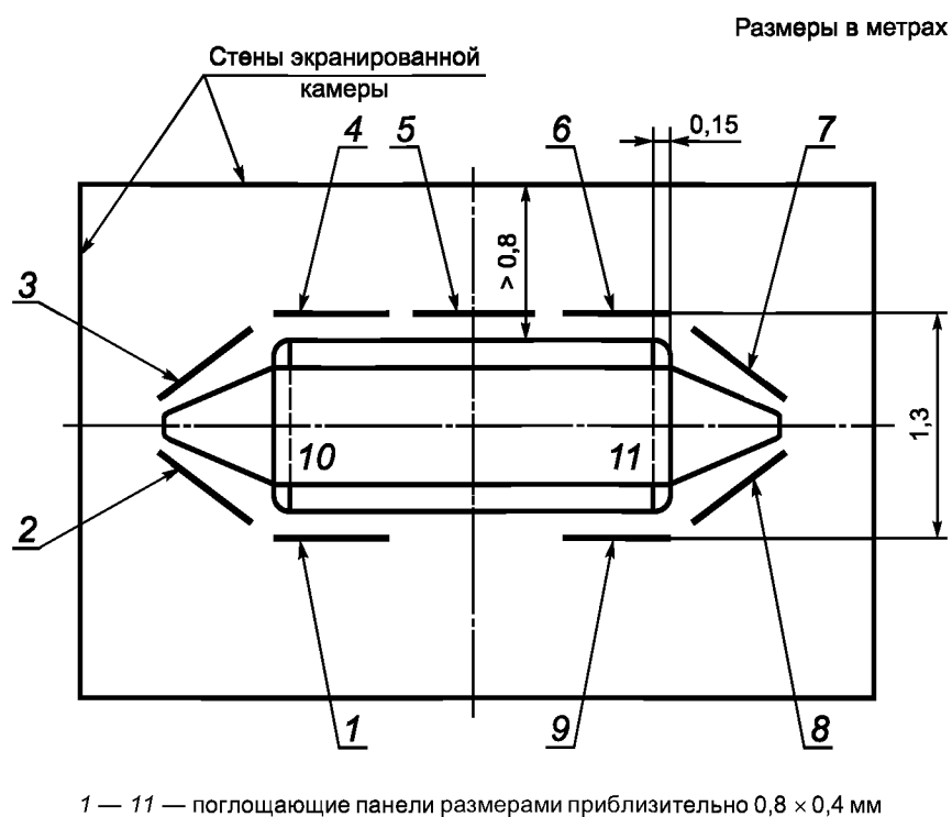
Рисунок 5 — Пример ТЕМ-устройства на базе открытой полосковой линии в комбинации с поглощающими панелями внутри экранированной камеры размерами 3 \times 3,5 м
