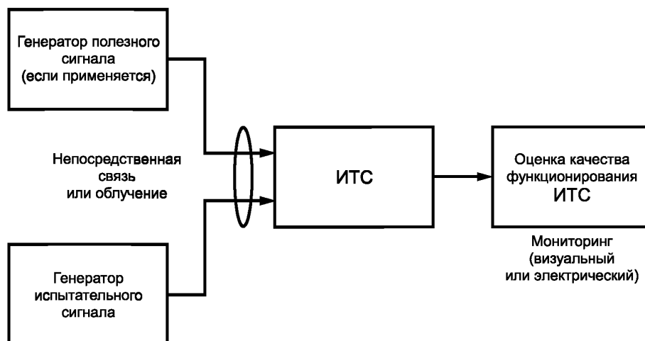
Рисунок 1 — Структурная схема измерения параметров помехоустойчивости
