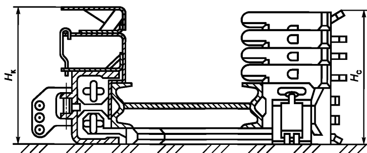
Рисунок 1 — Схема измерения высоты исполнительного органа установки и высоты конвейера
