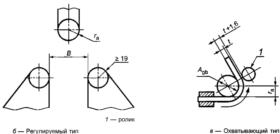
Рисунок 9, лист 2
