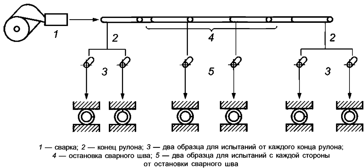
Рисунок 6 — Испытания на сплющивание
