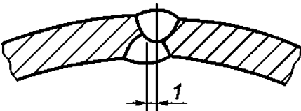
1 — смещение
