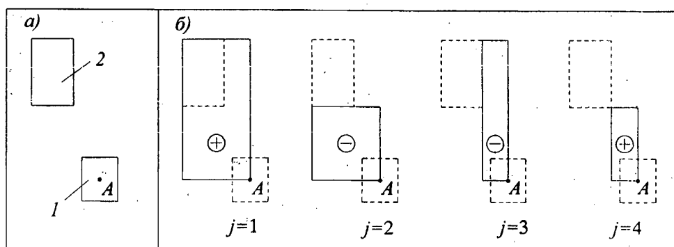
Рисунок 5.3 — Схема к определению вертикальных напряжений в основании рассчитываемого фундамента с учетом влияния соседнего фундамента методом угловых точек
