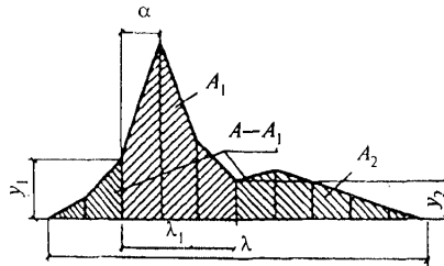
Рисунок К.2 – Часть линии влияния длиной \lambda_1 , включая ее вершину
