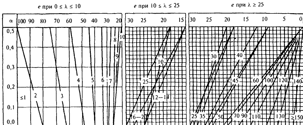
Рисунок К.1 – Коэффициент e в зависимости от \lambda и \alpha (длина заграждения \lambda , м, указана на графике)
