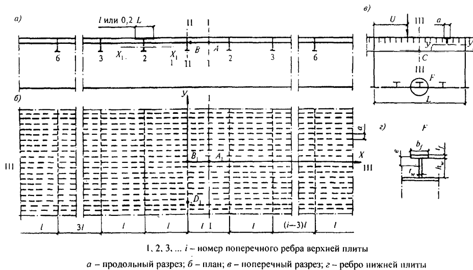
Рисунок Ш.1 — Коробчатое пролетное строение
