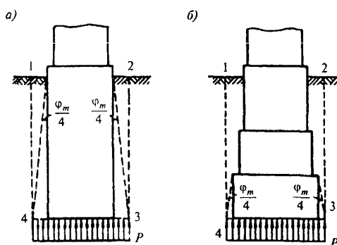
Рисунок 3.5 – Условный фундамент из опускного колодца
