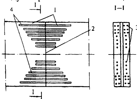
Рисунок 10.1 — Клеештыревой стык
