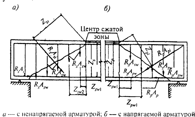
Рисунок 7.7 — Схема усилий в сечении, наклонном к продольной оси железобетонного элемента, при расчете его по прочности на действие изгибающего момента
