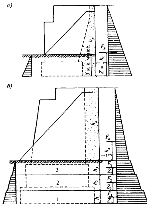
Рисунок Е.1 – Схема эпюр давления грунта на опоры моста для определения равнодействующей нормативного горизонтального (бокового) давления на опоры
