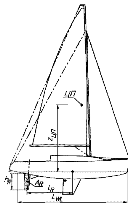
Рис. 3.1 Элементы парусного судна
