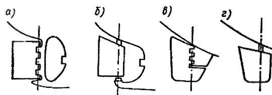
Рис. 2.1.6 Типы рулей:
