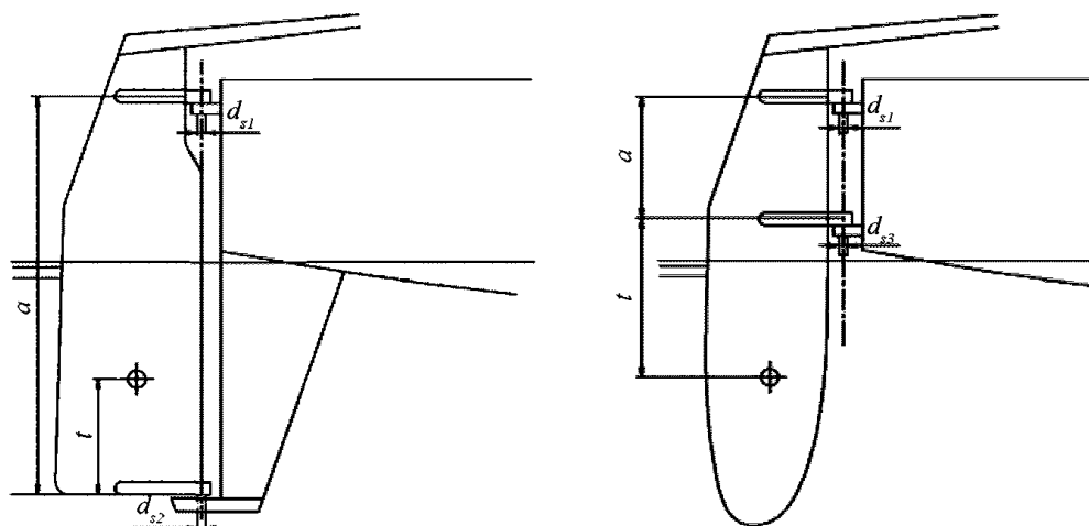
Рис. 2.5.3 Транцевые рули
