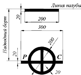
Рис. 6.2.2.1 Грузовая марка
