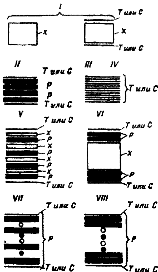
Рис. 6.1.1 Схемы армирования
