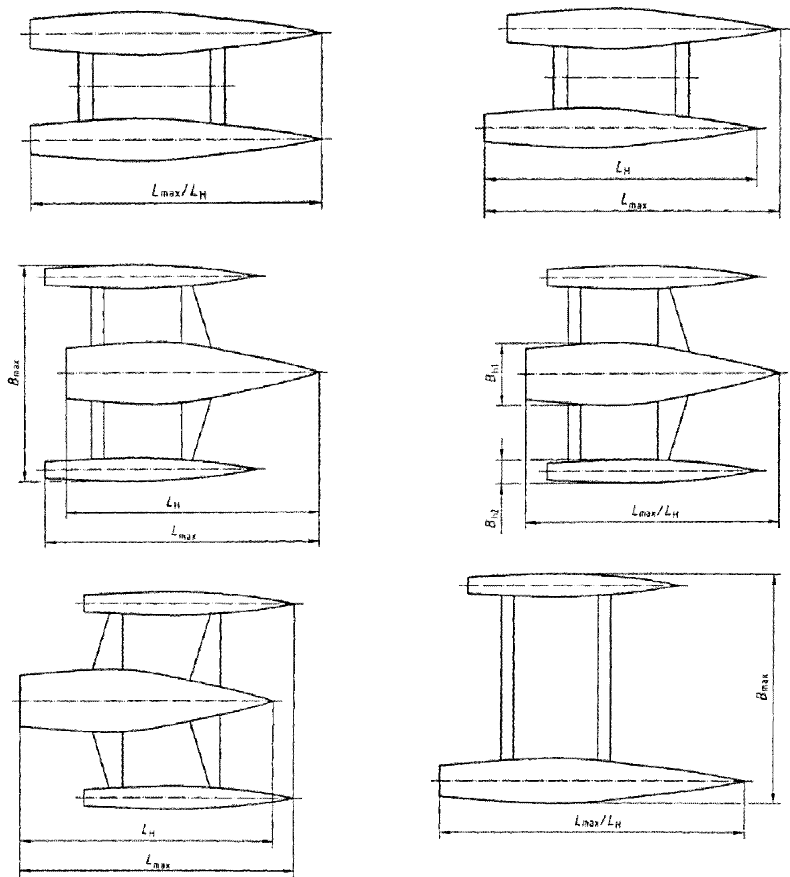
Рис. 3.2.3-3 Определение размерений L_{max} , L_H , B_{max} и B_H для многокорпусных судов
