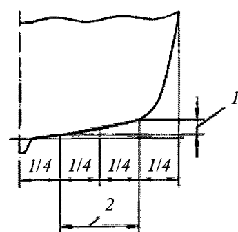
c) Выпуклое днище
