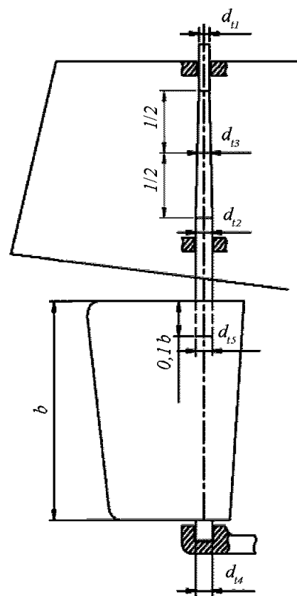
Рис. 2.4.3 Баллер руля.
