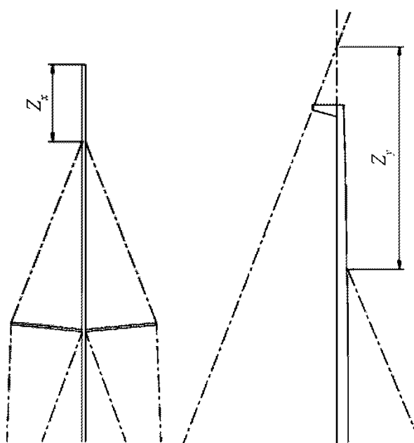
Рис. 5.4.1.6 Размеры топа мачты
