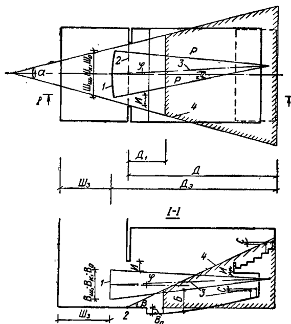
Рис. 1. Размещение зрительских мест, расположение и размеры экрана
