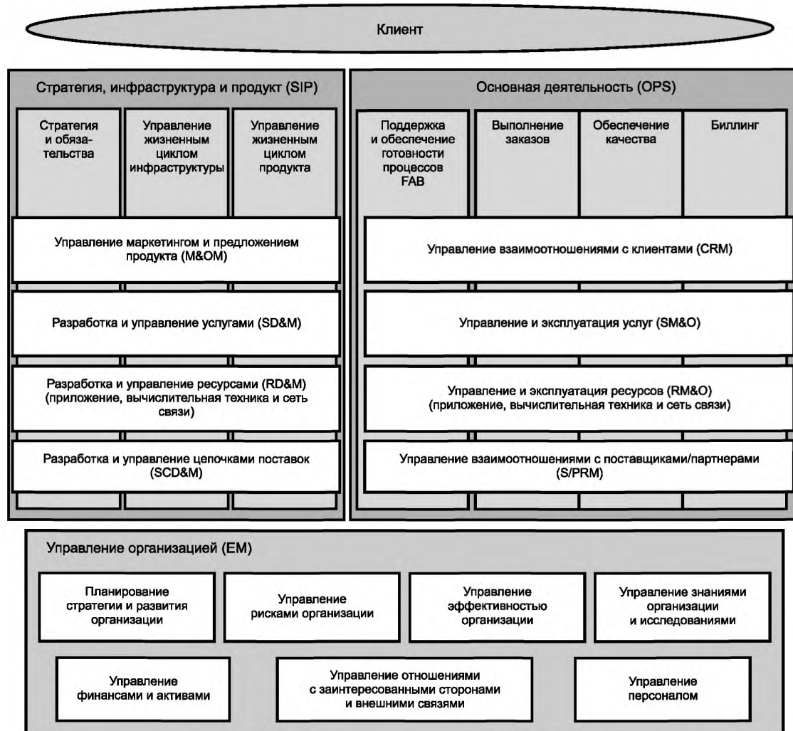
Рисунок 2 — Структура уровня 1 общей структуры бизнес-процессов еТОМ
