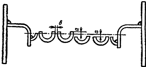
Рис. 2. Установка съемных деталей тарелок
