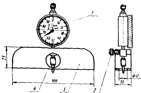
1—индикатор; 2—винт; 3—колодка; 4—наконечник индикатора.
