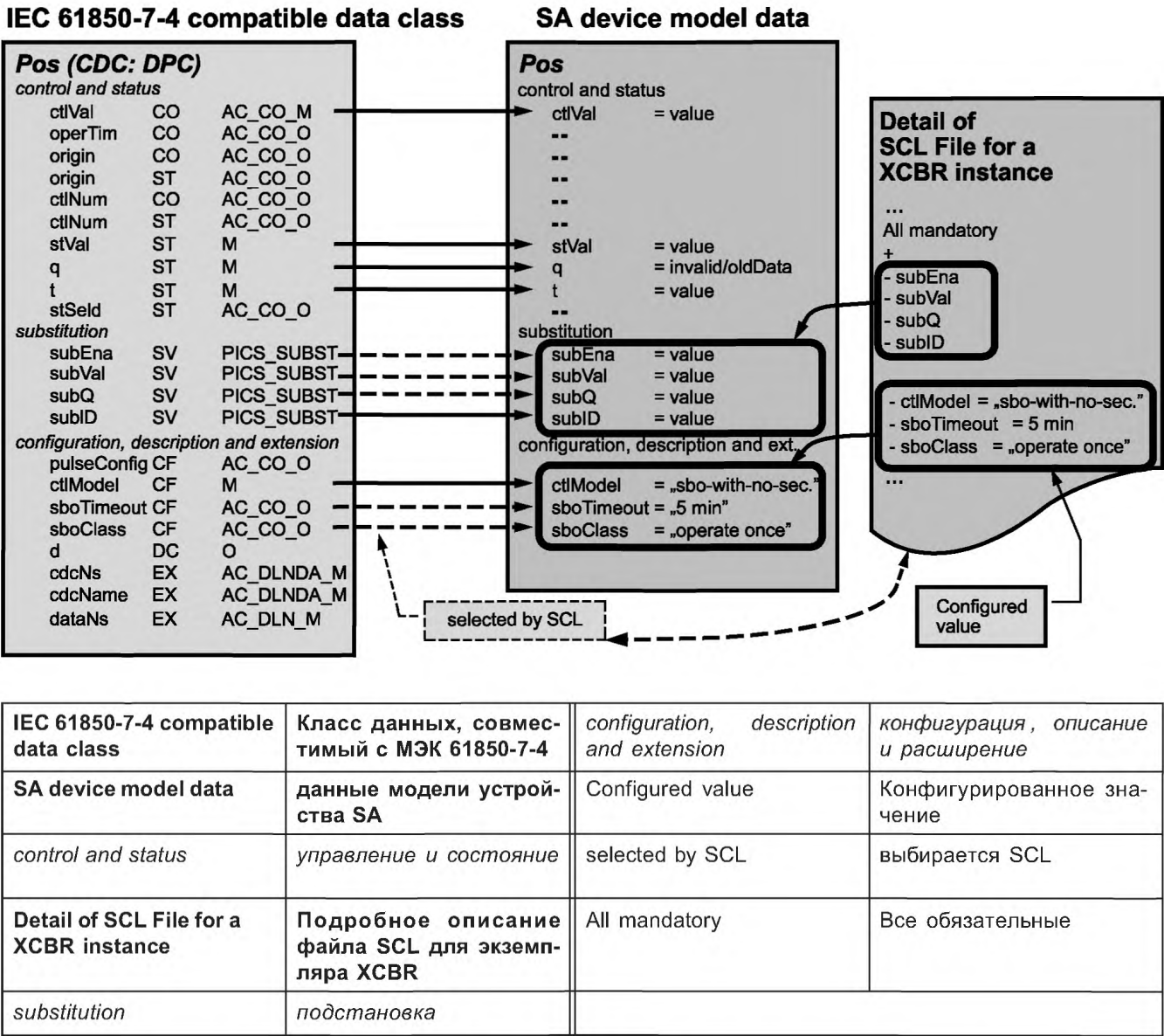
Рисунок С.2 — Использование SCL для данных (концептуальное представление)
