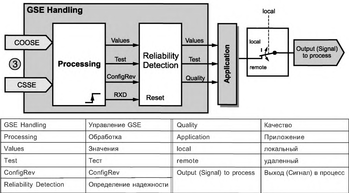
Рисунок 15 — Модель выхода GSE (концептуальное представление)
