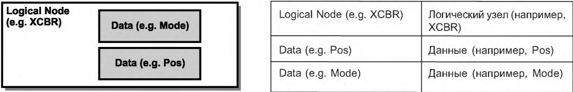
Рисунок 29 — Логические узлы и данные (МЭК 61850-7-2)
