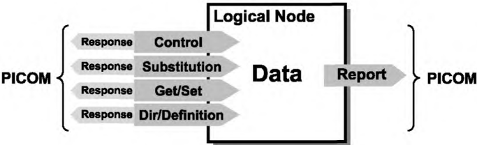
Рисунок 32 — Логические узлы и PICOM
