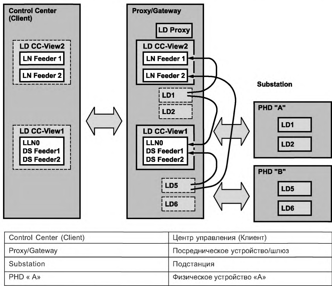
Рисунок D.1 — Прямая связь (упрощенное представление)
