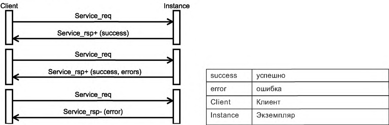
Рисунок 65 — Диаграмма последовательностей
