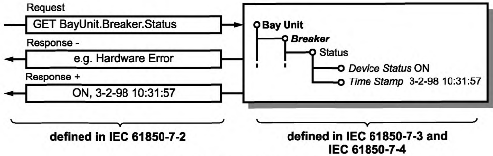
Рисунок 44 — Пример сервиса, лист 1
