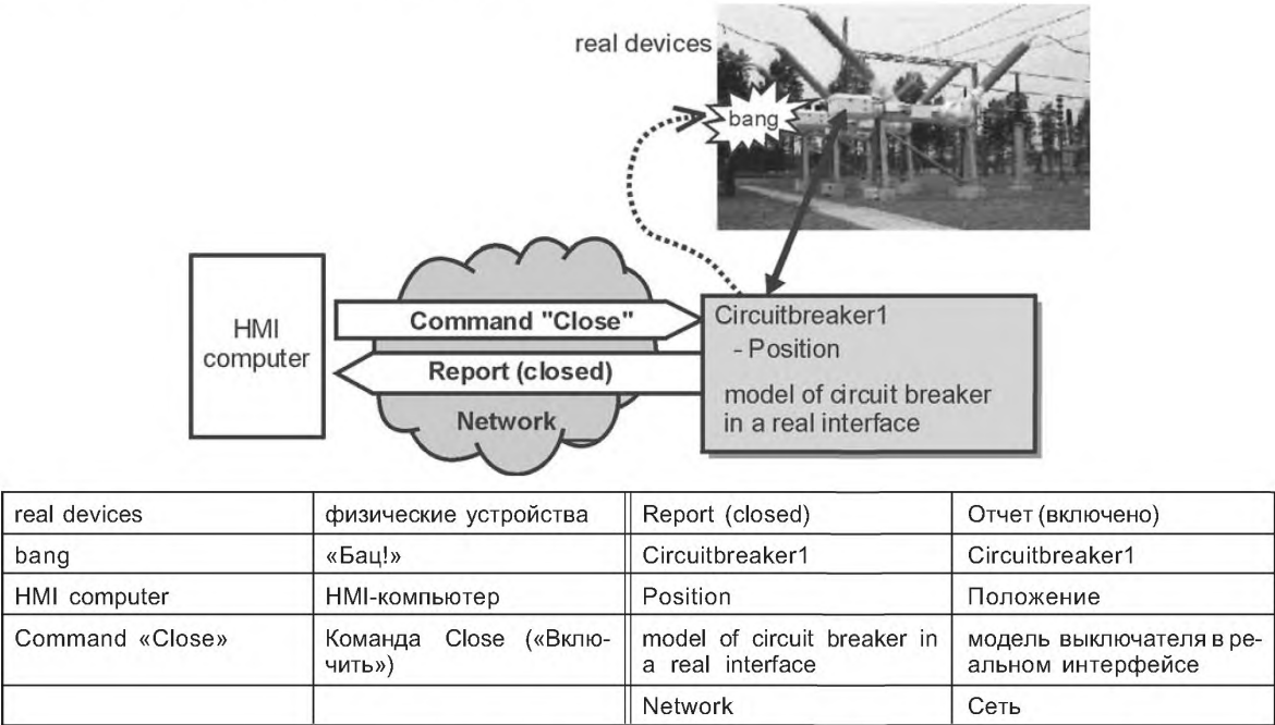
Рисунок 28 — Физические устройства
