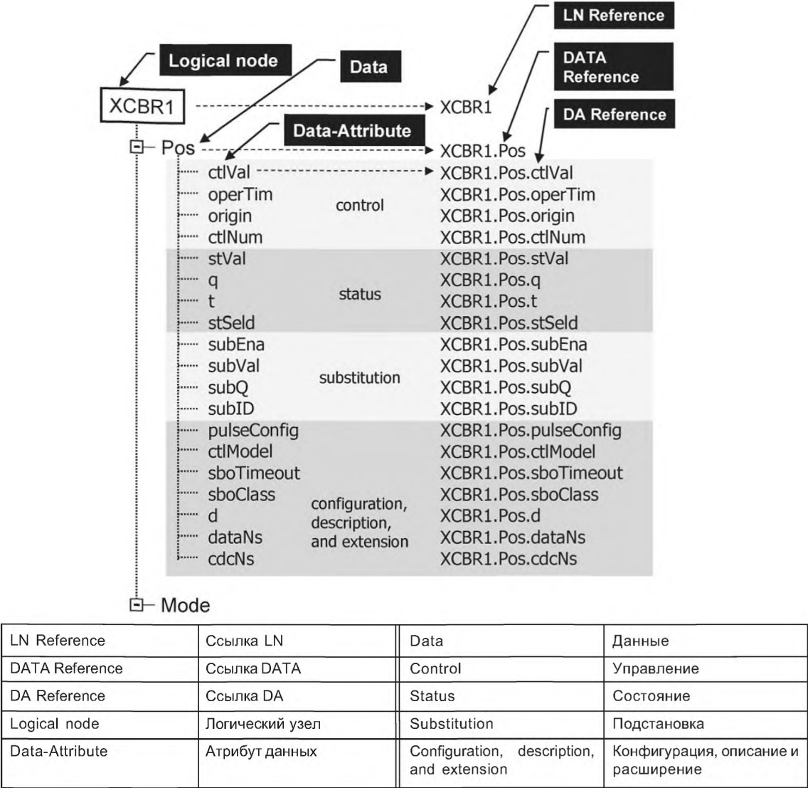
Рисунок 10 — Информация XCBR1 в виде дерева
