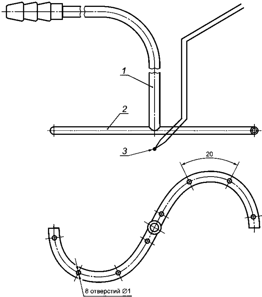
Рисунок 10 — Пробоотборник для отбора проб продуктов сгорания для испытательных дымоходов диаметром D < 100 мм
