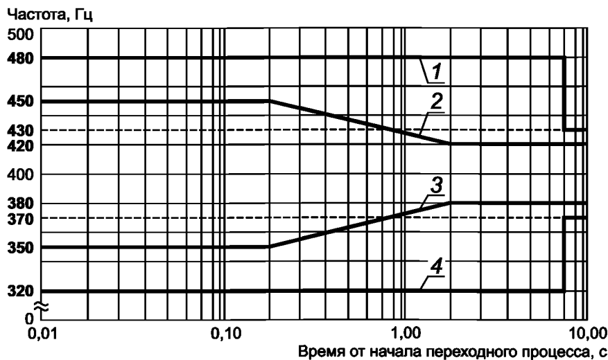
1 и 4 — верхний и нижний пределы ненормальной переходной частоты; 2 и 3 — верхний и нижний пределы нормальной переходной частоты
