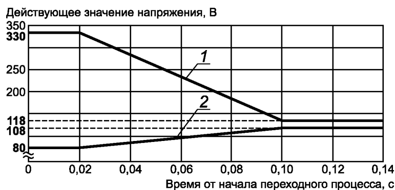
1 — верхний предел действующего значения напряжения; 2 — нижний предел действующего значения напряжения
