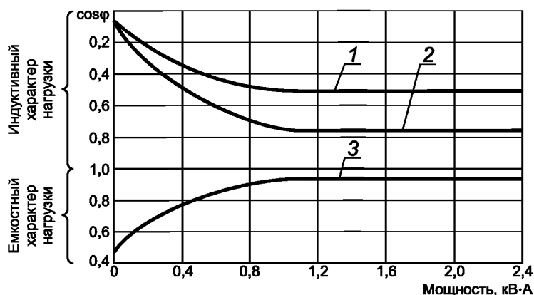
1 — асинхронные электродвигатели; 2 — индуктивная нагрузка; 3 — емкостная нагрузка
