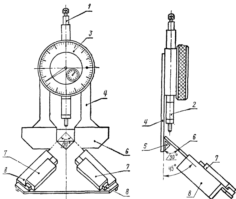
1 — стержень измерителя; 2 — съемный наконечник стержня диаметром 3 или 10 мм; 3 — индикатор часового типа ИЧ10 класса 1 по ГОСТ 577—68; 4 — хомут; 5 — призма; 6 — пластина; 7 — направляющие; 8 — салазки.
