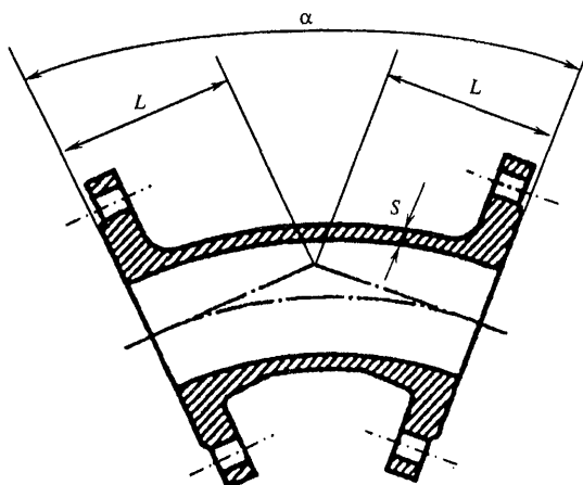
Рисунок Б.12 – Отвод фланцевый
