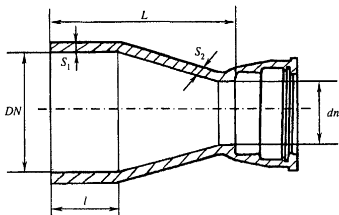
Рисунок Б.13 – Переход раструб – гладкий конец
