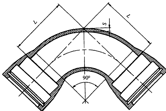
Рисунок Б.9 – Колено раструбное
