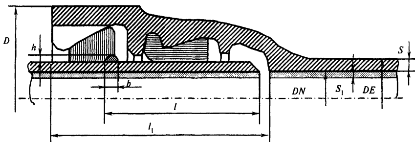
Рисунок Б.1 – Раструбное соединение типа «R»
