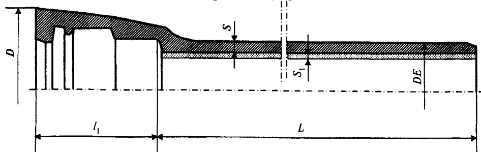
Рисунок А.1 – Труба раструбная под соединение «TYTON»
