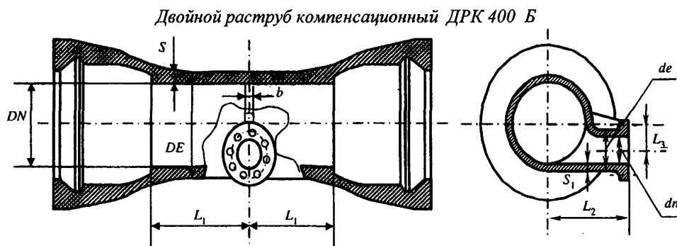
Рисунок Б.22 – Выпуск раструбный
