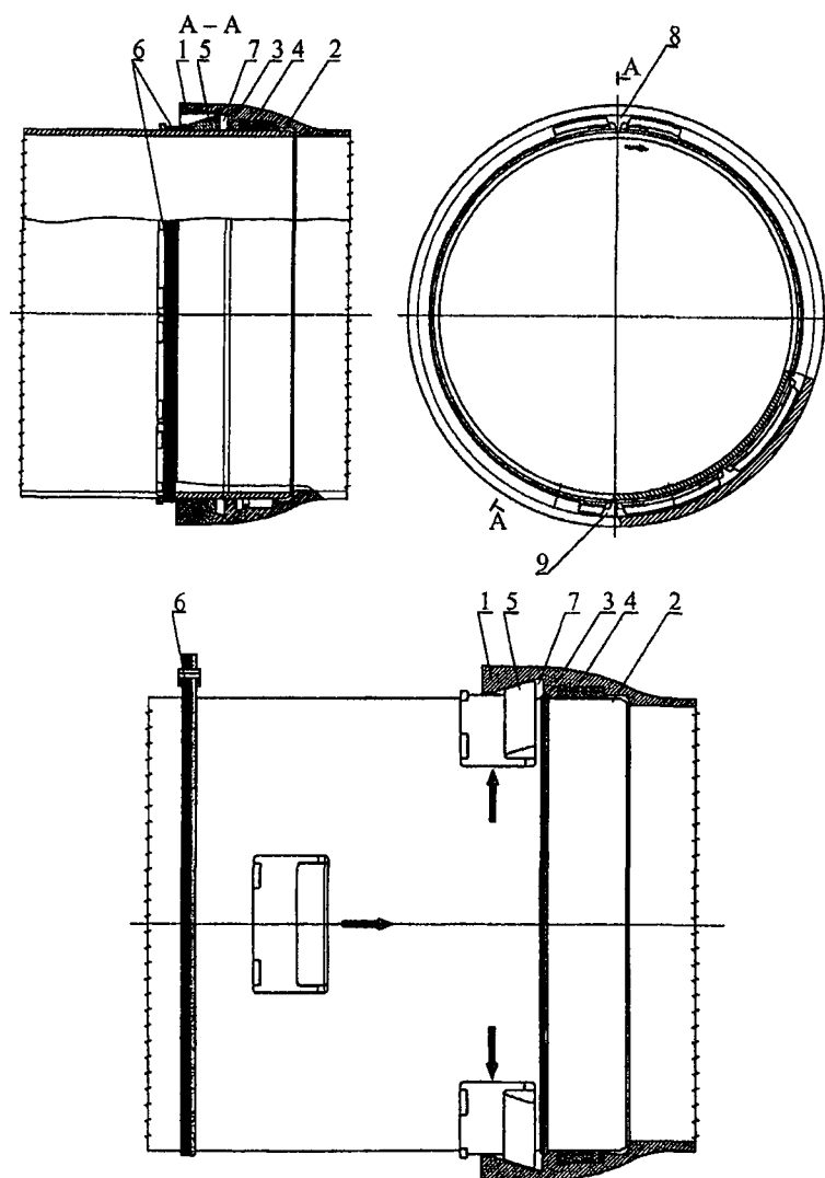
Рисунок 10.2 – Замковые соединения типа «RJS»
