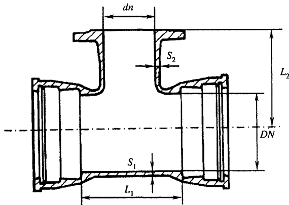
Рисунок Б.4 – Тройник раструб-фланец
