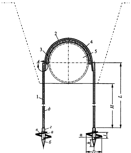
1 – металлические винтовые анкеры; 2 – силовой пояс; 3 – футеровочный мат; 4 – прокладки; 5 – труба; а – сердечник; б – наконечник; в – винтовая лопасть; г – оголовок; д – стержень
