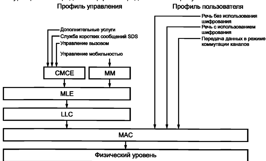
Рисунок 4.6 — Архитектура радиоинтерфейса TETRA V + D (TMO) ( U_m )
