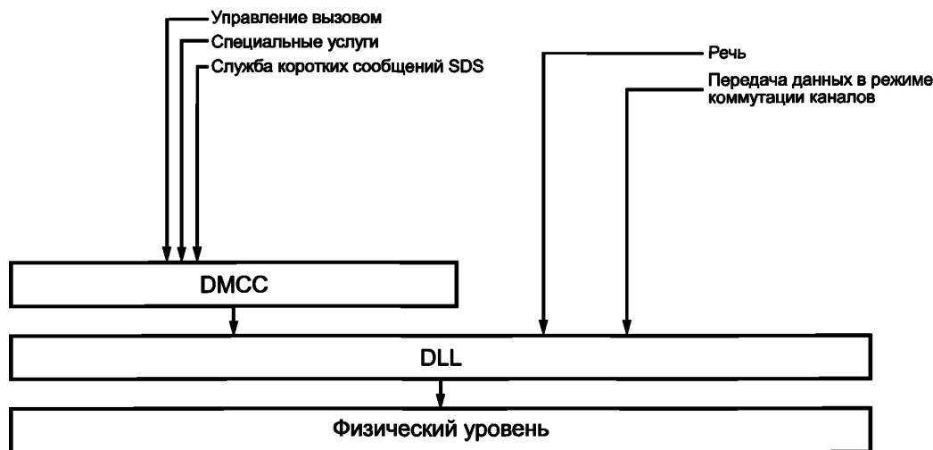
Рисунок 4.7 — Архитектура радиоинтерфейса TETRA DMO
