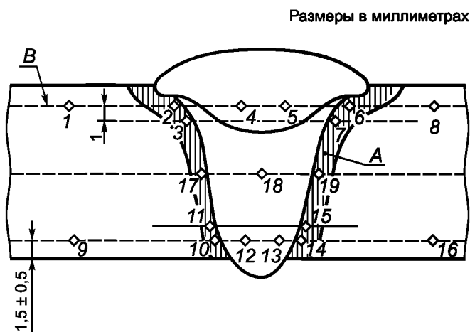
А — зона термического влияния (видима после травления); В — линии обследования
