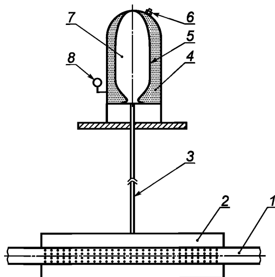
1 — перфорированный центральный трубопровод; 2 — предкамера; 3 — присоединительный патрубок; 4 — газ под давлением; 5 — эластичная разделительная перегородка (оболочка); 6 — штуцер для заправки газа; 7 — полость для рабочей среды; 8 — манометр
