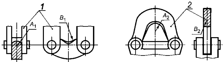
1 — скоба талевого блока; 2 — штроп крюка Рисунок 1 — Талевый блок и штроп крюка
