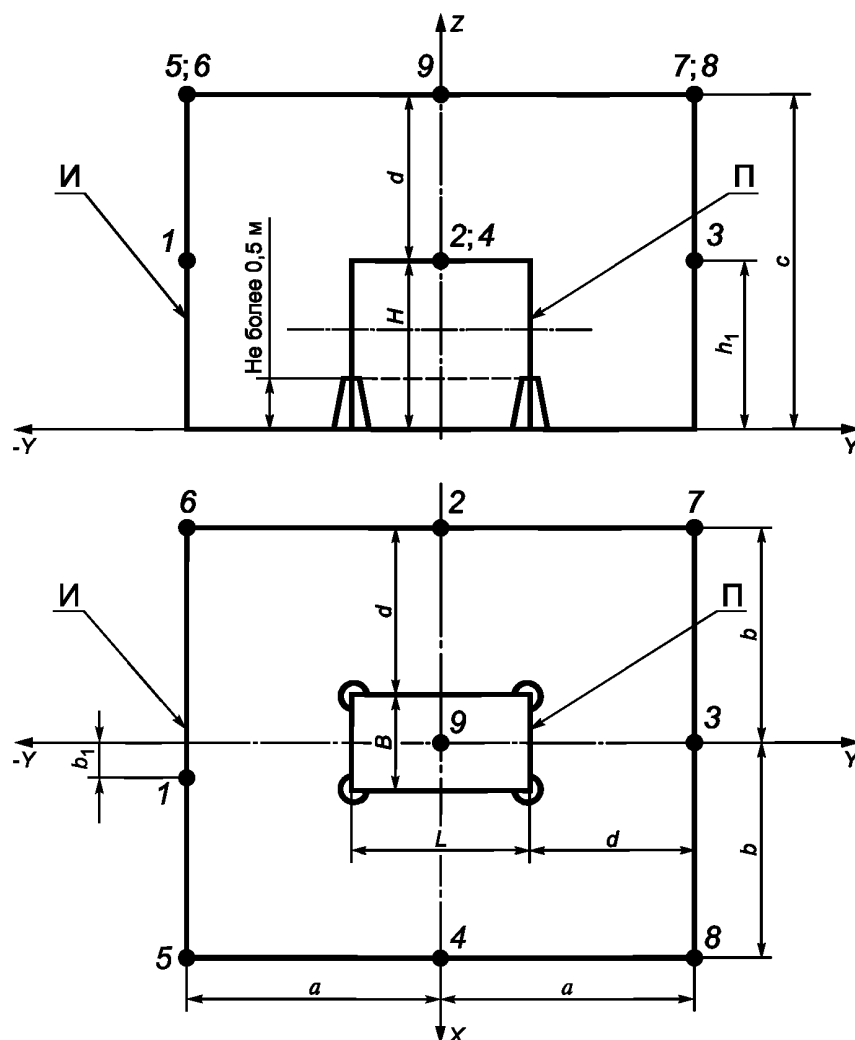
И — измерительная поверхность; П — поверхность параллелепипеда; 1—9 — точки измерения; B , L , H — размеры параллелепипеда; a , b , c — характеристические размеры измерительной поверхности; d — расстояние от поверхности параллелепипеда П до измерительной поверхности И
