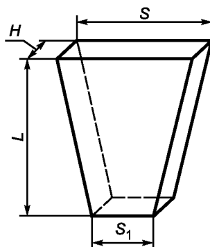
Рисунок 2 — Трапецеидальный двусторонний клин (стенное изделие)
