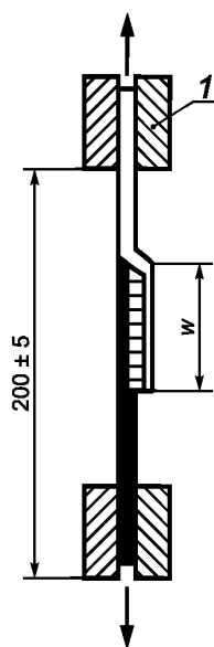
Рисунок 1 — Схема закрепления образца
