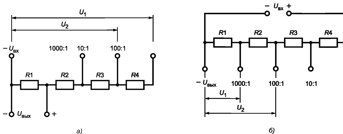
Рисунок 4 — Схема проверки делителя напряжения методом опорного напряжения
