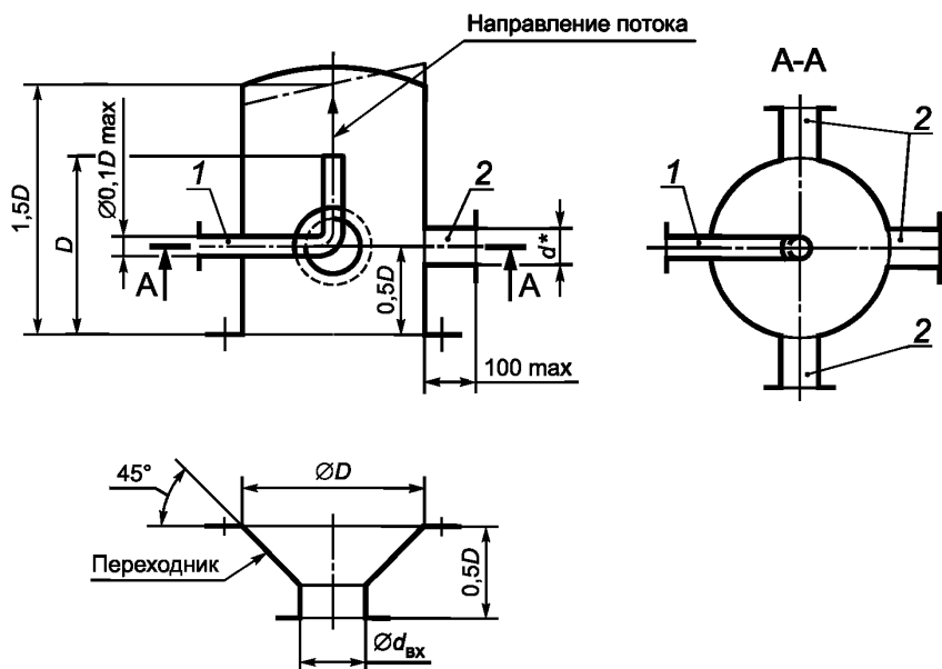
1 — напускная трубка; 2 — патрубок для подсоединения вакуумметра
