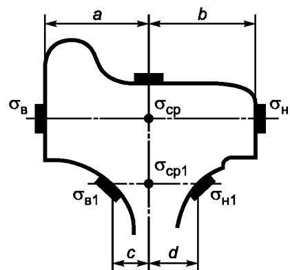
Рисунок А.6 — Схема приведения к плоскости круга катания ( \sigma_{cp} и \sigma_{cp1} ) напряжений замеренных ( \sigma_B , \sigma_H , \sigma_{B1} , \sigma_{H1} ) на боковых поверхностях обода (бандажа) и приободной части диска
