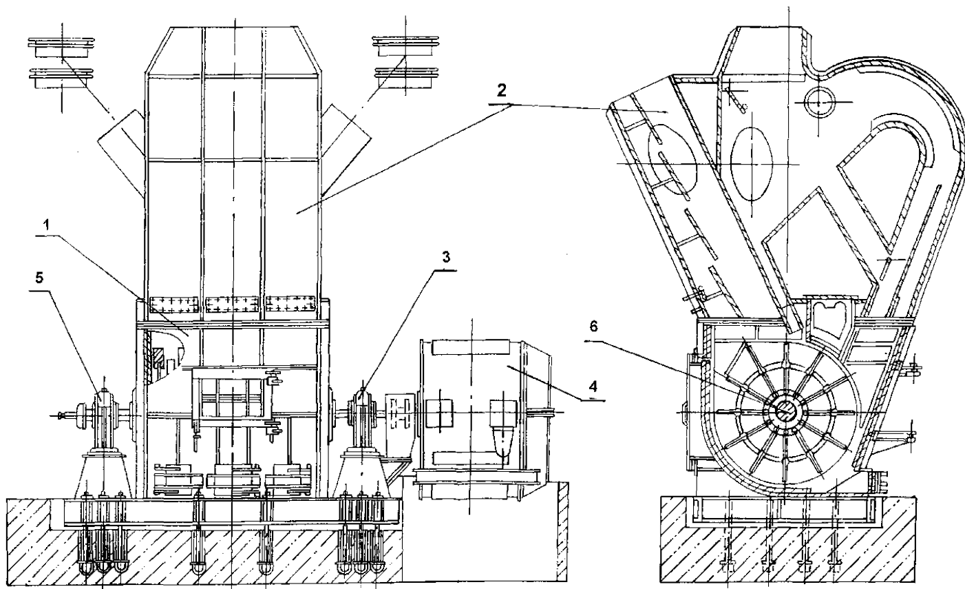
1— корпус мельницы; 2— сепаратор; 3— подшипник опорно-упорный; 4— электродвигатель; 5— подшипник опорный; 6— ротор
