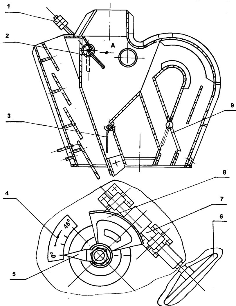
1— противовес; 2— лопатка; 3— лопатка; 4— шкала указателя; 5— стрелка; 6— маховичок; 7— тяга; 8— сектор червячный; 9— лопатка.
