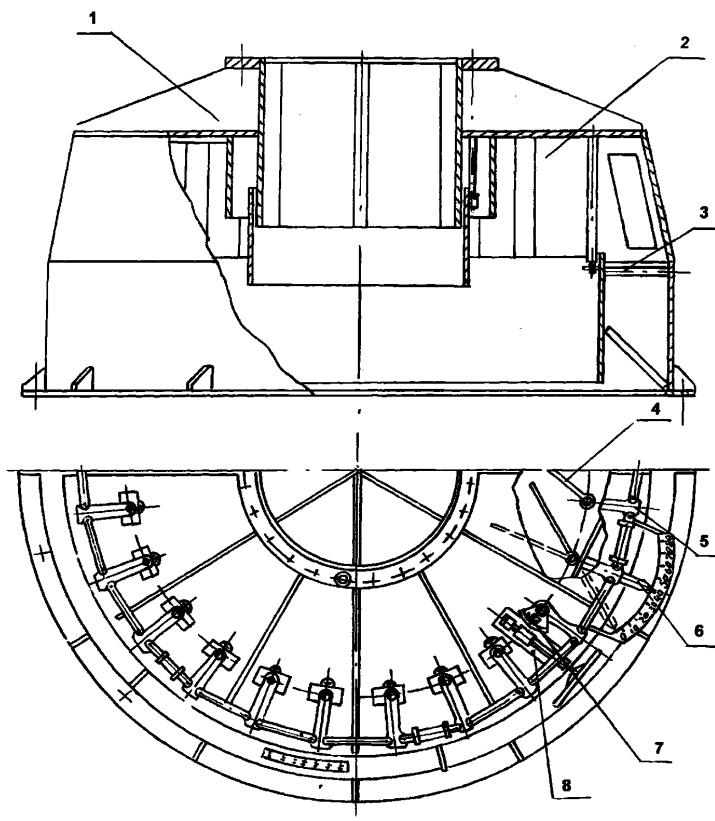
1– корпус сепаратора; 2– лопатка; 3– растяжка; 4– лопатка; 5– рычаг; 6– стрелка; 7– червячный сектор; 8– червяк
