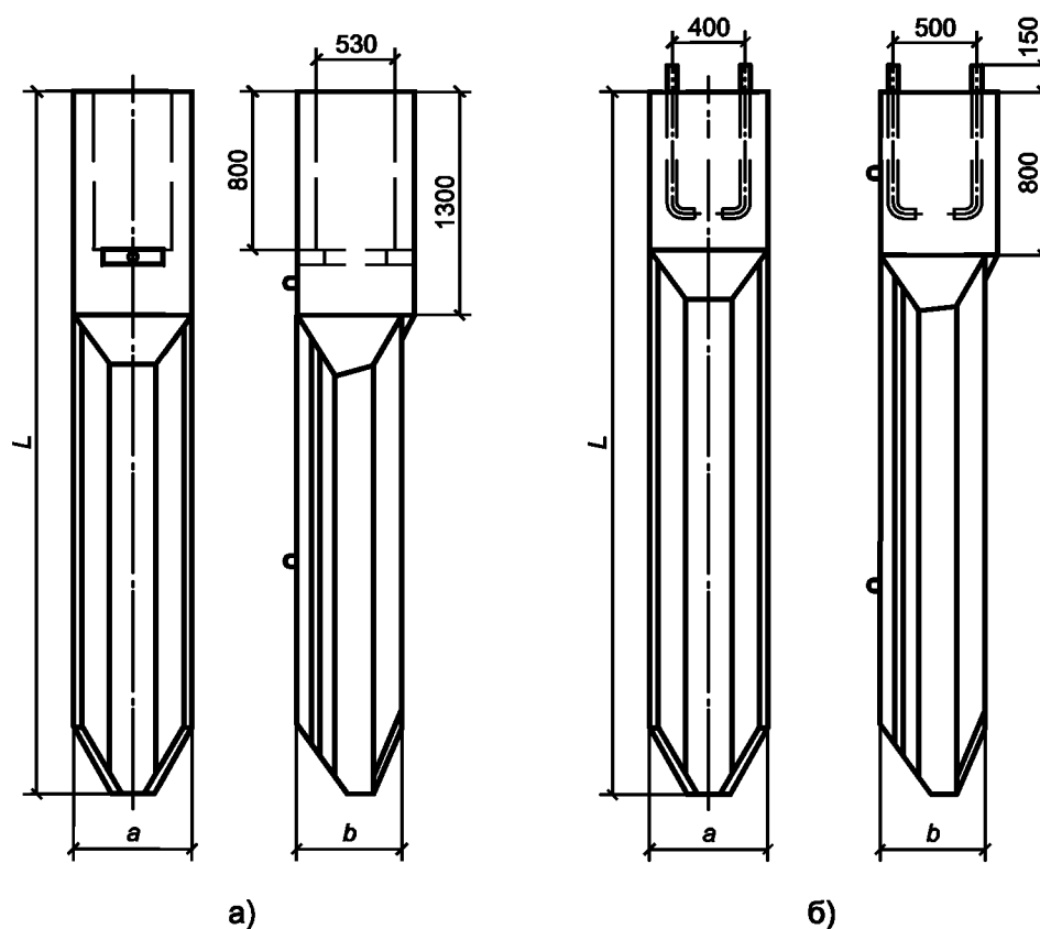
Рисунок 1 — Трехлучевые фундаменты:
