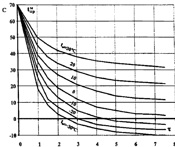
Рисунок Б.3 – Температура мазута в цистернах при транспортировке в зависимости от температуры окружающего воздуха и времени нахождения в пути
