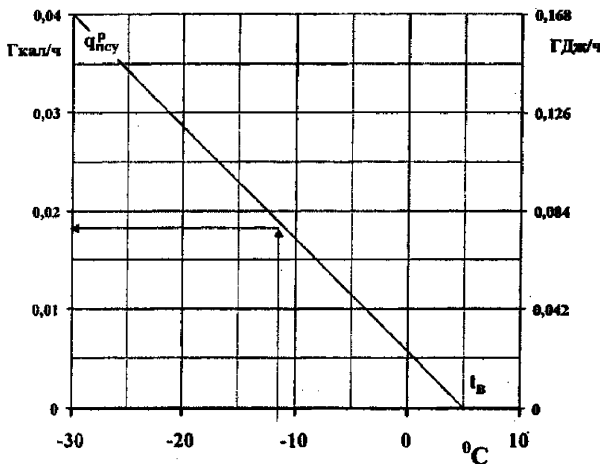
Рисунок Б.8 Нормы удельного расхода тепла на поддержание одного парового «гусака» приемно-сливного устройства в резерве ( q_{\text{плс}}^{\text{р}} ), учитываемые при эксплуатации
