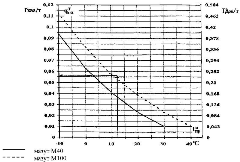
Рисунок Б.2 – Нормы удельного расхода тепла при сливе мазута ( q_{ссл}^T ), учитываемые при эксплуатации ХЖКТ
