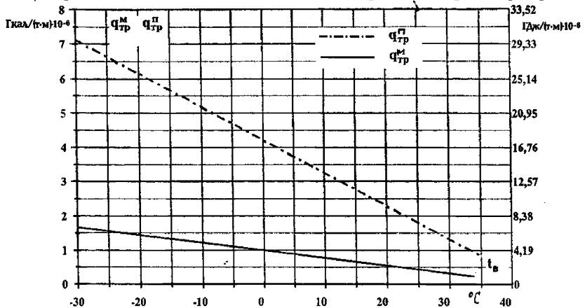
Рисунок Б.5 – Нормы удельного расхода тепла при транспортировке мазута ( q_{гр}^м ) и пара ( q_{гр}^п ) по трубопроводам, учитываемые при проектировании и эксплуатации ХЖКТ
