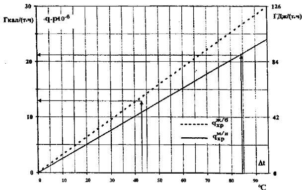
Рисунок Б.6 – Нормы удельного расхода тепла при хранении мазута в железобетонных ( q_{ж/б} ), металлических с изоляцией ( q_{м/и} ) емкостях, учитываемые при эксплуатации
