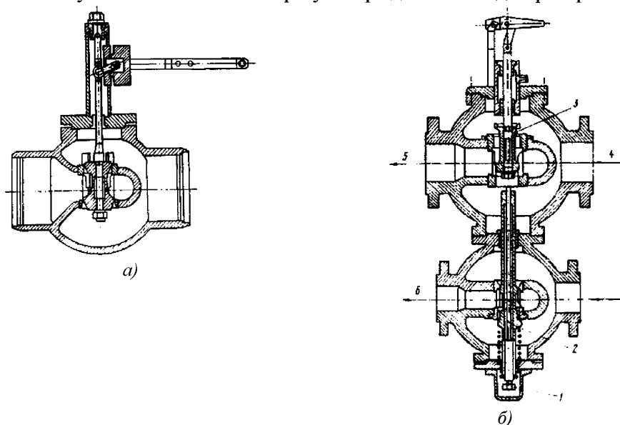
Рисунок И1.9 – Клапаны регулятора давления в деаэраторе
