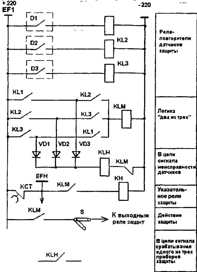
Рисунок Э.14 – Электрическая схема защиты по схеме «два из трех»
