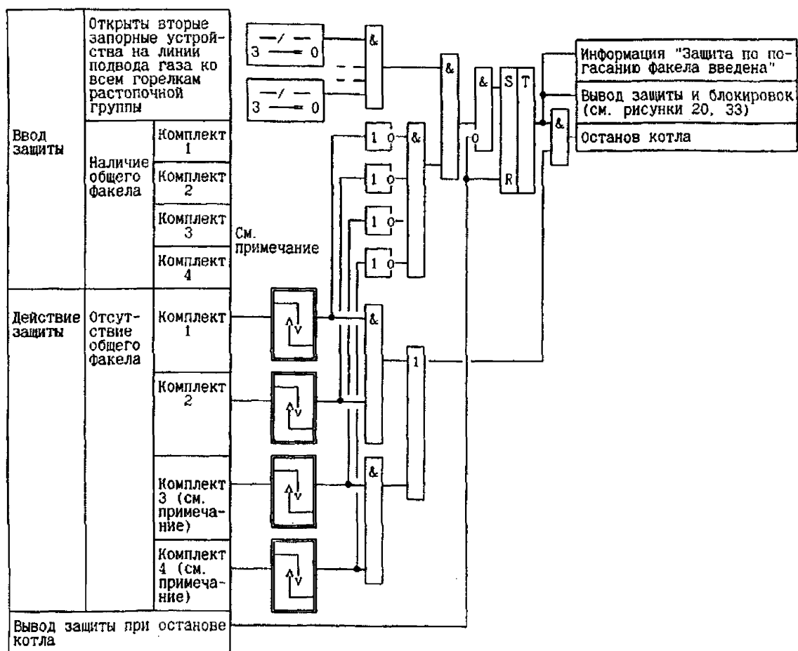
Рисунок Ф.6 - Защита по погасанию общего факела в топке Газовый котел без ПЗК у горелок
