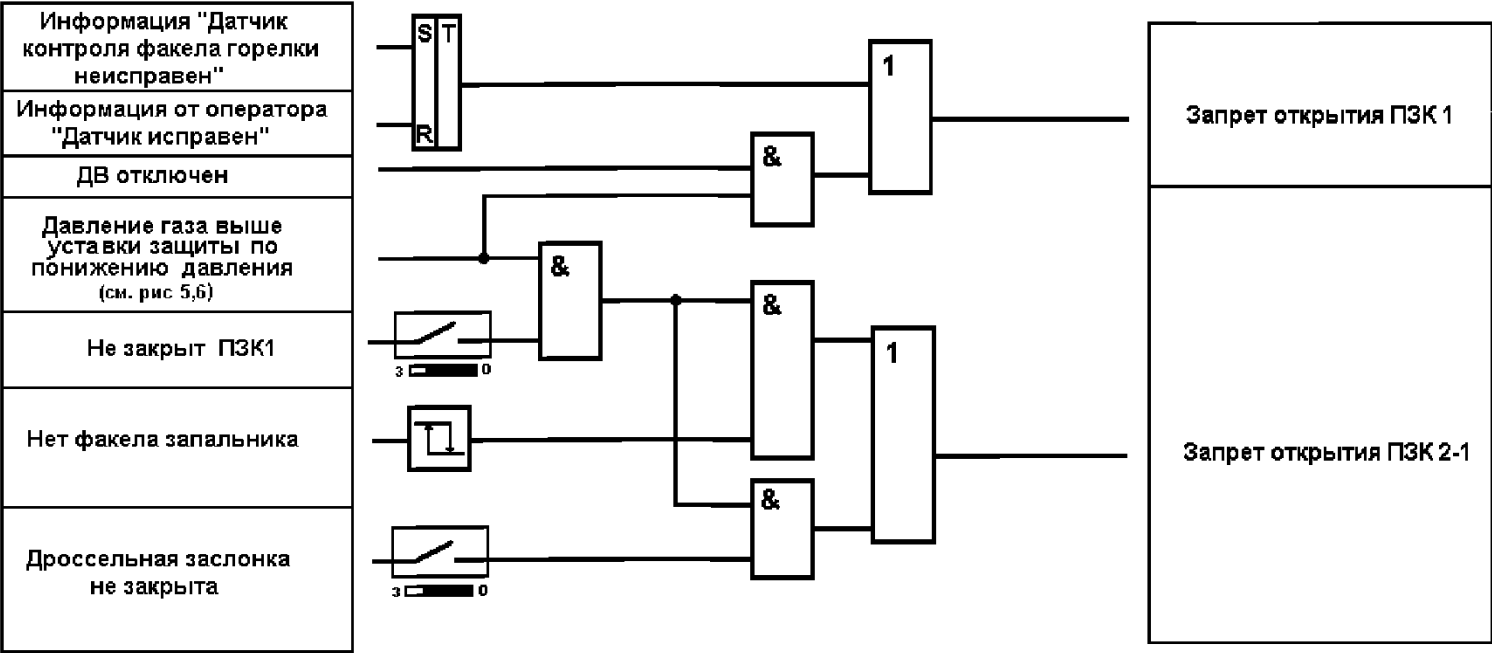
Рисунок Х.15 – Алгоритм блокировок растопочной горелки с БГ-13 при работе на газе
