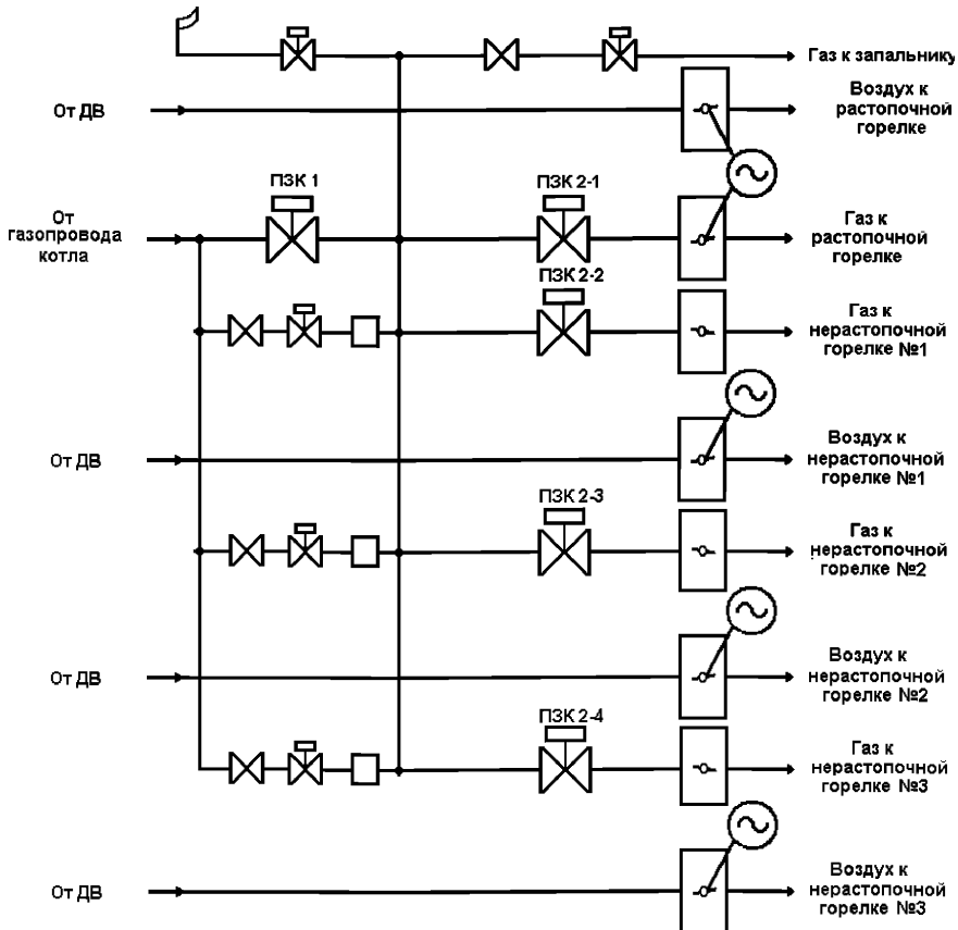
Рисунок Ш.1а – Схема газо- и воздухопроводов БГ с тремя нерастопочными горелками
