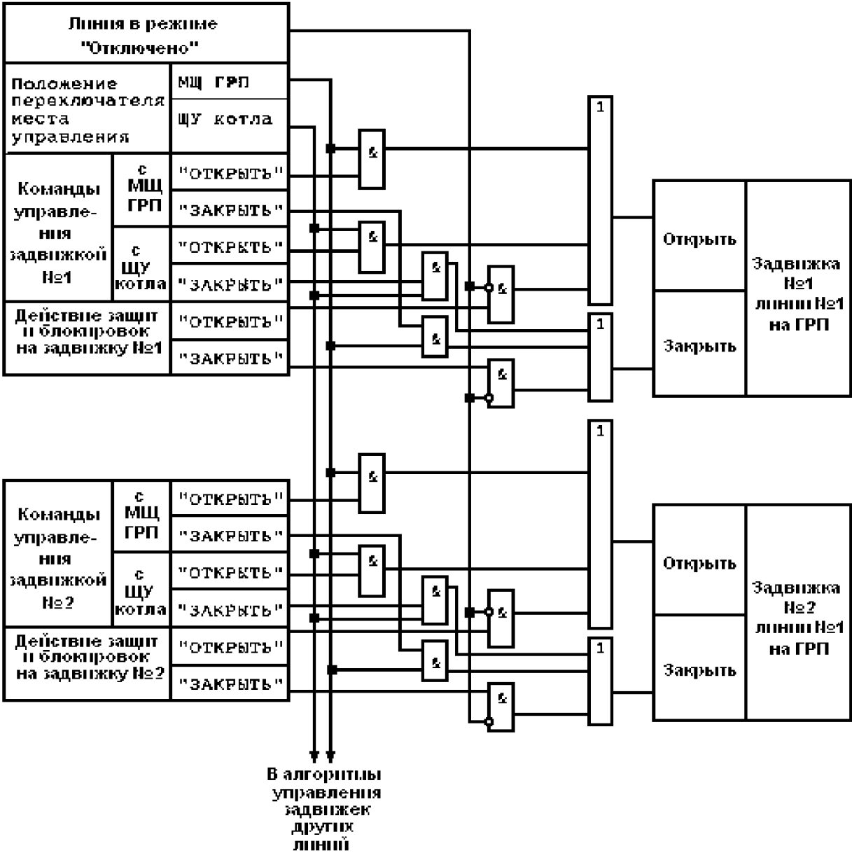
Примечание – Схема дана для задвижек одной линии ГРП. Рисунок У.6 – Структурная схема блокировок при управлении арматурой ГРП с двух мест
