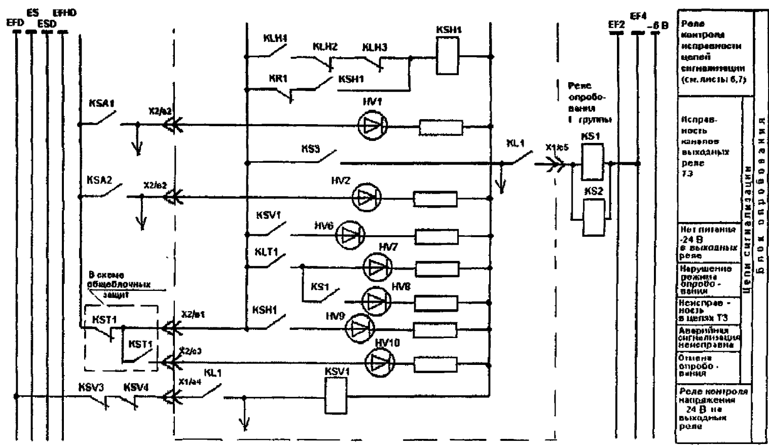
Рисунок Э.22 – Организация электрической схемы опробования ТЗ на УКТЗ (лист 5)
