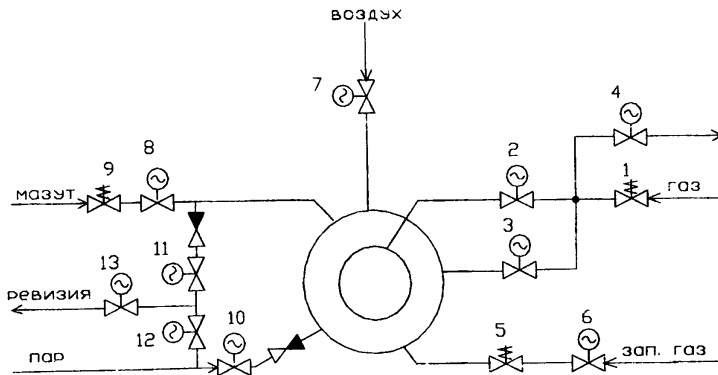
Рисунок Ц.1 – Схема газомазутной горелки
