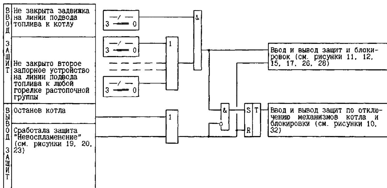
Рисунок Ф.2 - Ввод защит при начале растопки и вывод после останова котла.
