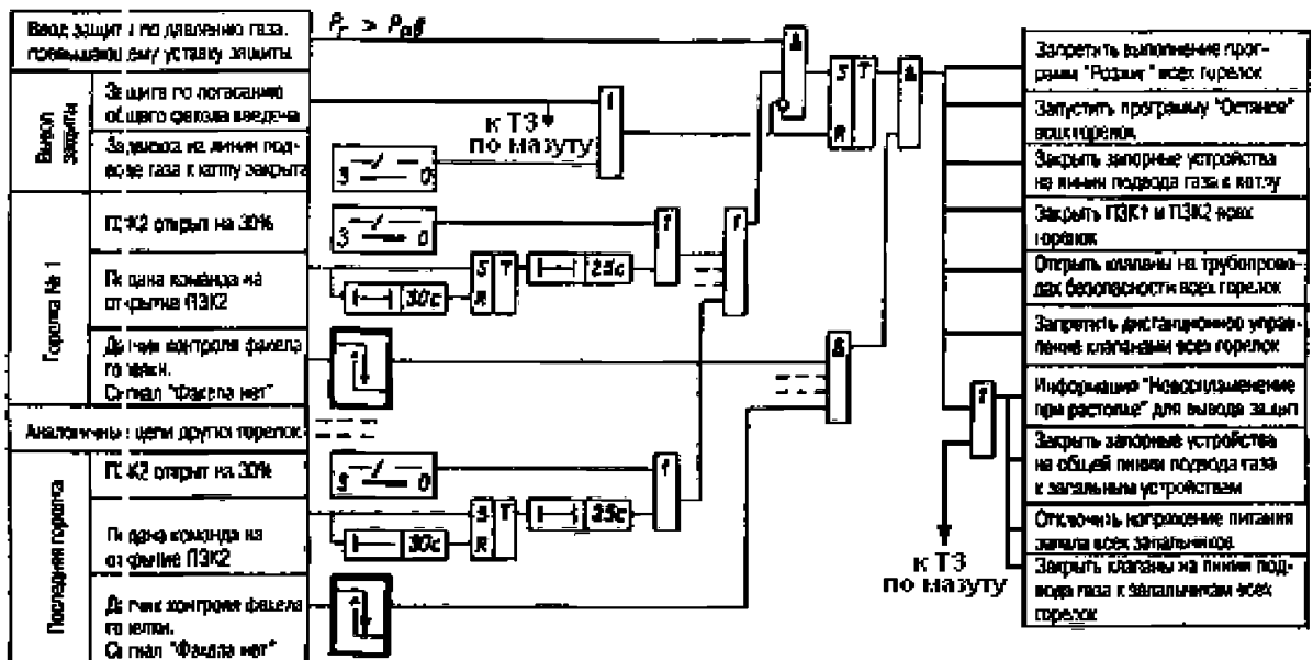
Рисунок Ц.4 - Алгоритм защиты «Невоспламенению первой или погасание факела всех газовых горелок при растопке газомазутного котла на газе»
