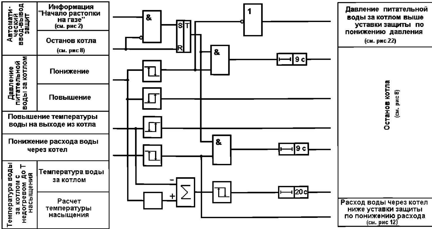
Рисунок Х.3 – Алгоритмы защит водяного тракта
