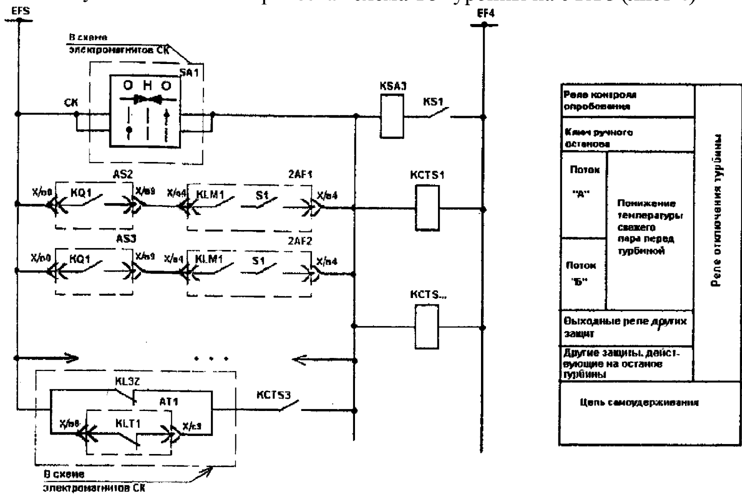
Рисунок Э.18 – Электрическая схема ТЗ турбины на УКТЗ (лист 5)
