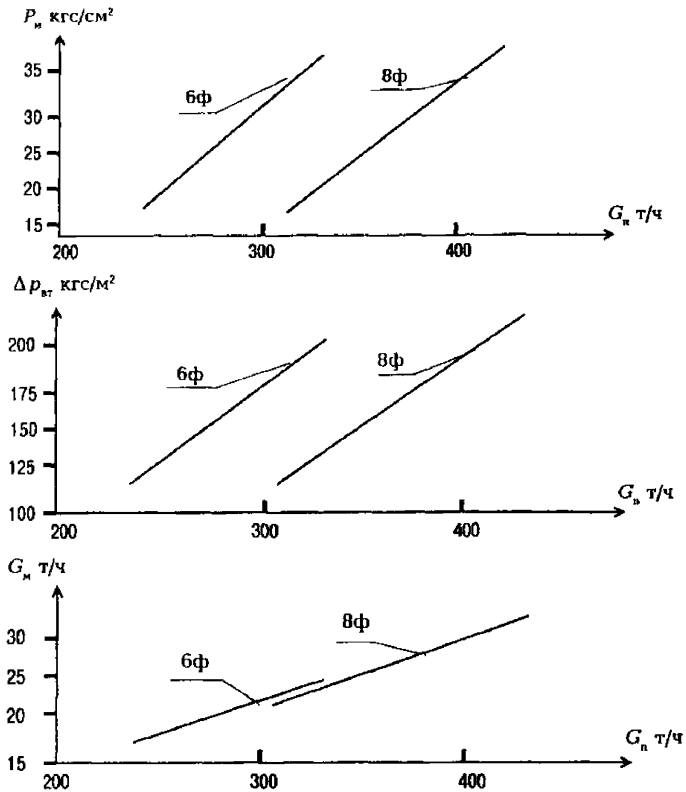
Рисунок Н.2 – Статические характеристики давления мазута ( p_n ), перепада давлений «воздух - топка» ( \Delta p_{\text{вт}} ) и расхода мазута ( G_n ) котла БКЗ-420-140 при работе на шести и восьми форсунках (ф)
