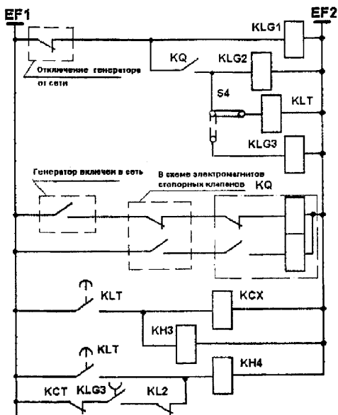
Рисунок Э.12 – Электрическая схема общецлочных защит (лист 2)
