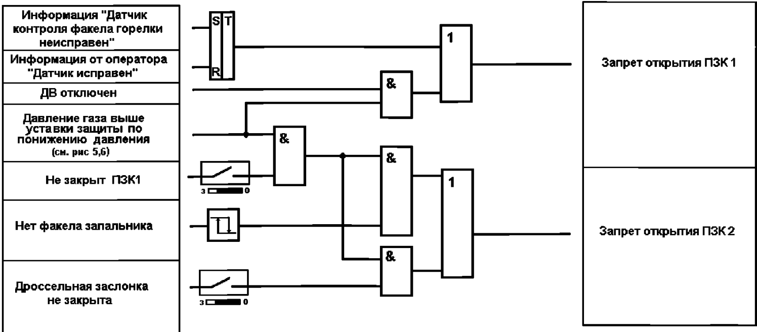
Рисунок Х.14 – Алгоритм блокировок растопочной горелки с БГ-8 при работе на газе
