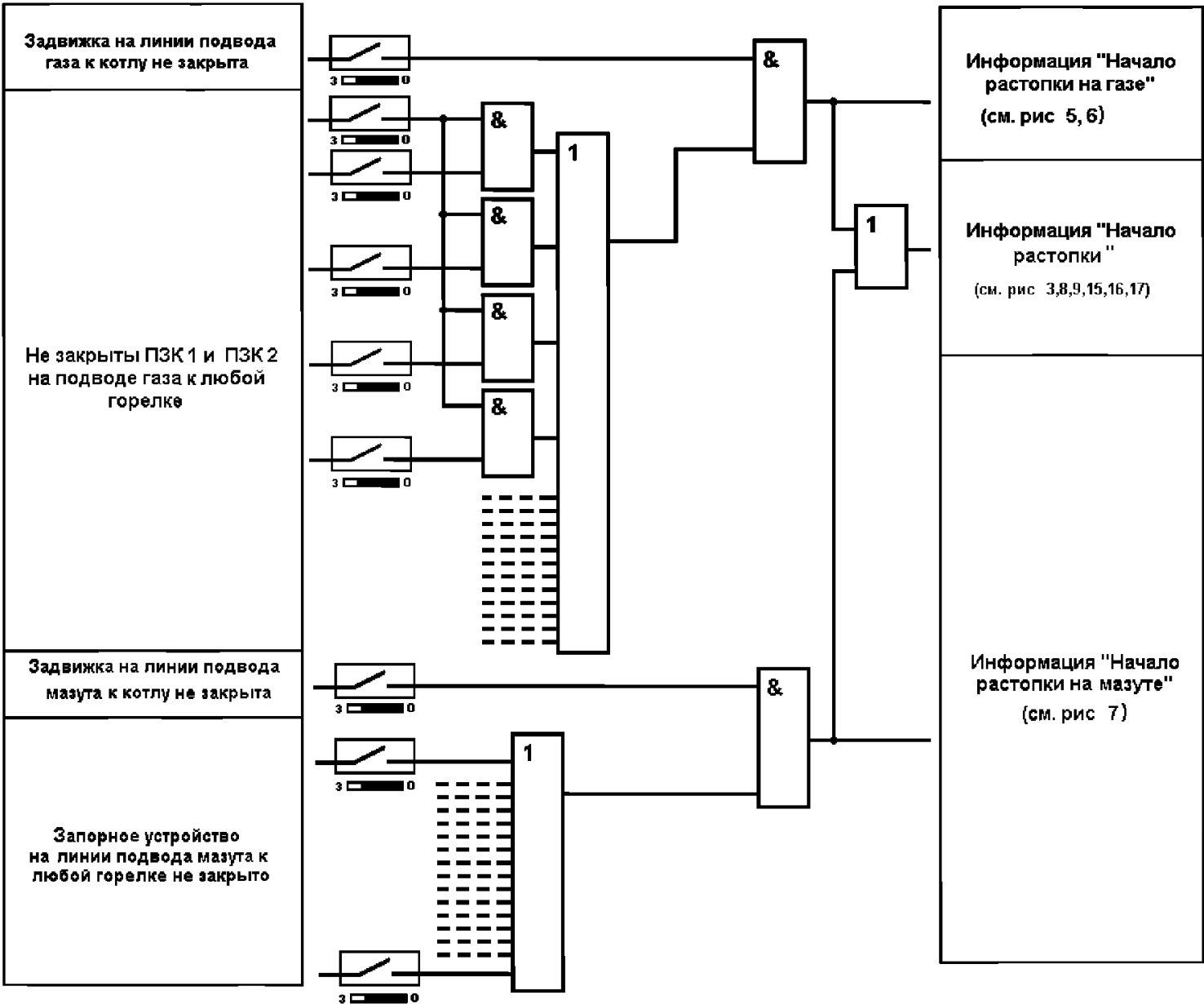
Рисунок Ш.2 – Алгоритмы формирования информации «Начало растопки»
