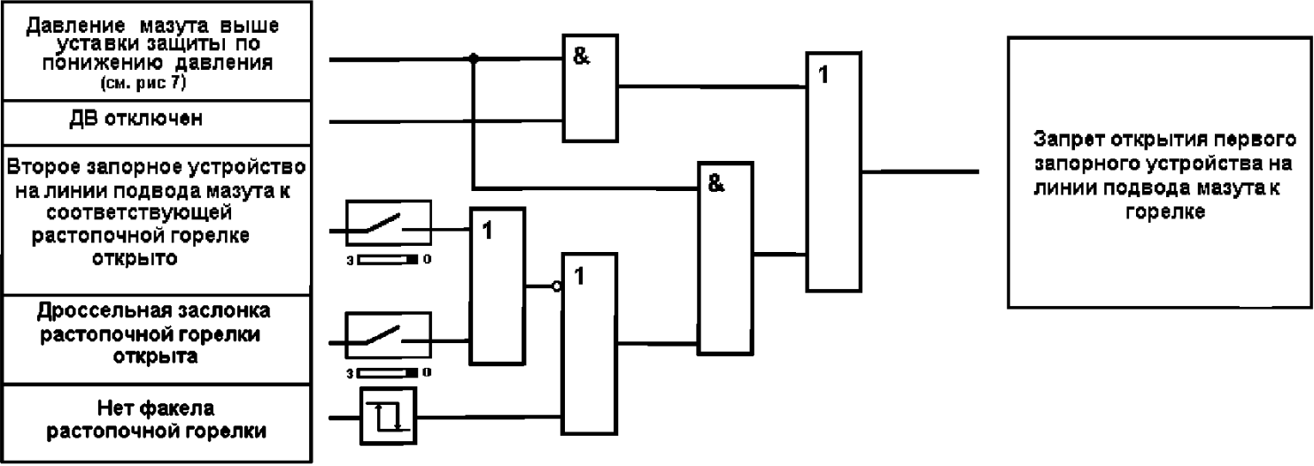
Рисунок Х.18 – Алгоритм блокировок растопочной горелки при работе на мазуте
