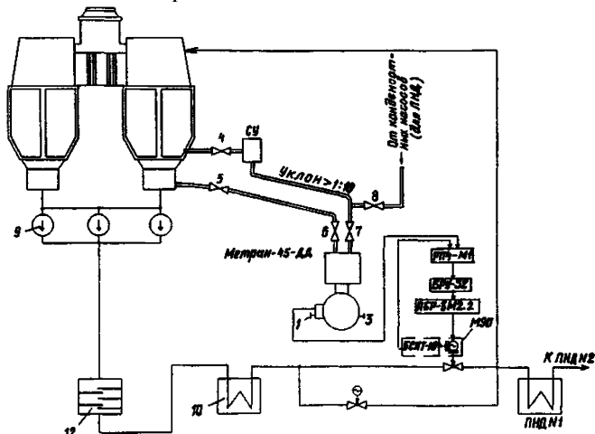
Рисунок И1.6 - Схема регулирования уровня в конденсаторе турбины
