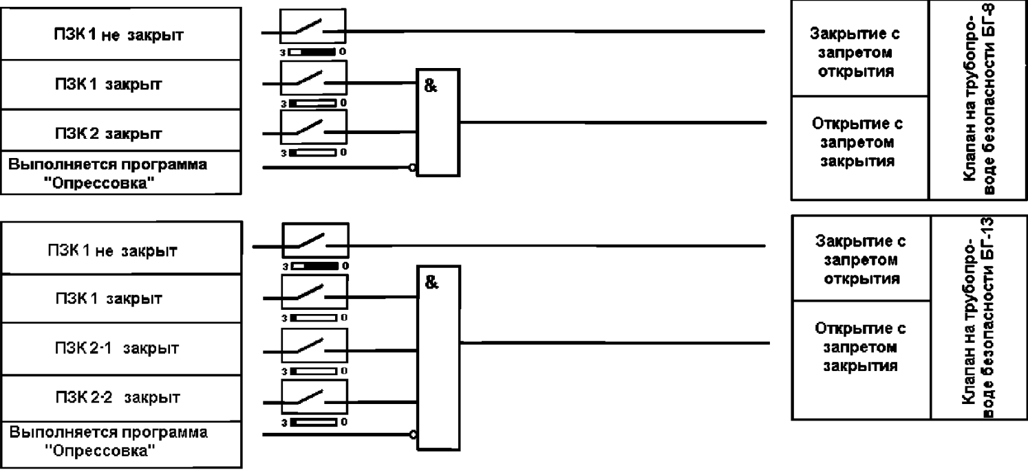
Рисунок Х.19 – Алгоритмы. блокировок клапана на трубопроводе безопасности газовой горелки
