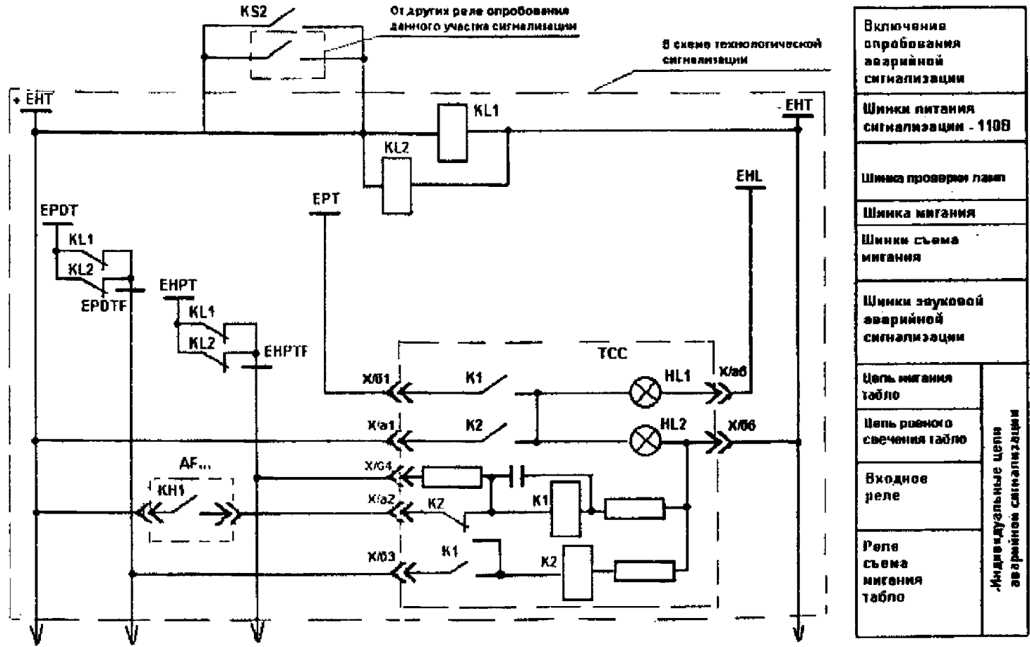
Рисунок Э.22 – Организация электрической схемы опробования ТЗ на УКТЗ (лист 6)
