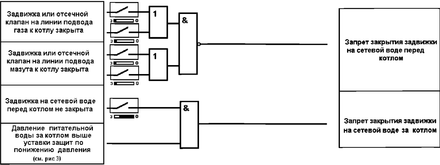
Рисунок Ш.25 - Алгоритмы блокировок задвижек на сетевой воде
