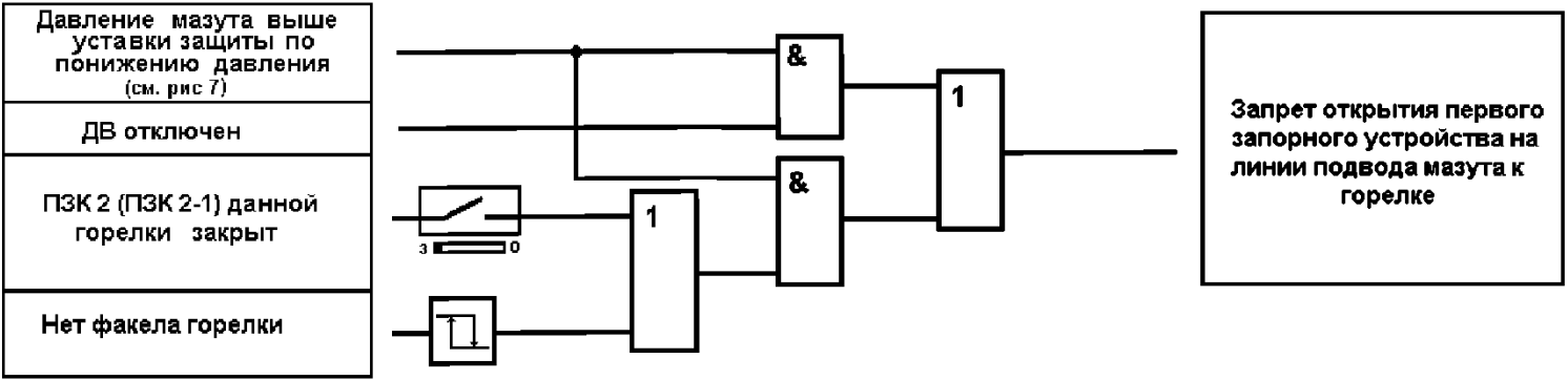
Рисунок Х.16 – Алгоритм блокировок растопочной горелки при работе на мазуте
