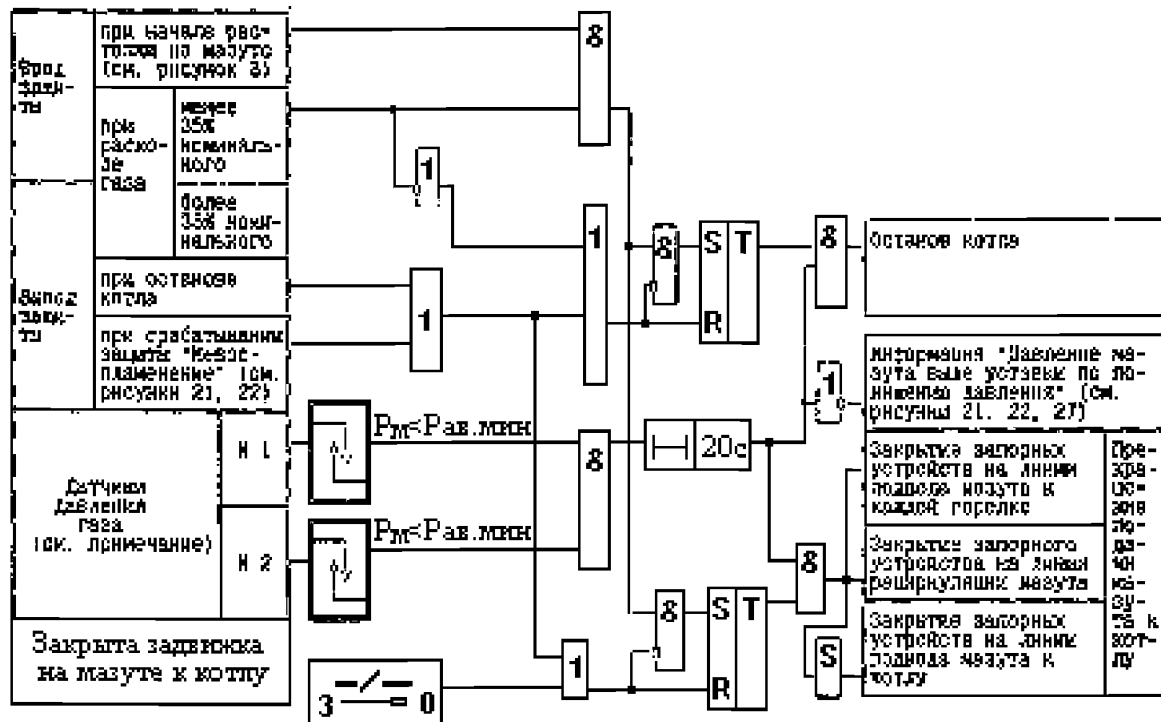
Рисунок Ф.16 - Защита по понижению давления мазута
