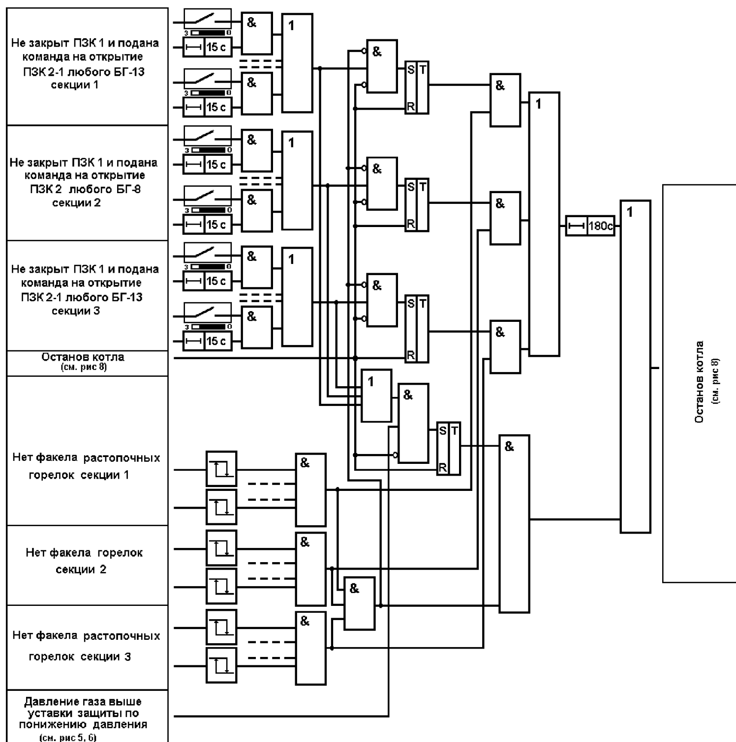
Рисунок Х.4 – Алгоритмы защит «Невоспламенение первой или погасание факела всех горелок в любой секции топки» и «Невоспламенение первой или погасание факела всех горелок в котле»
