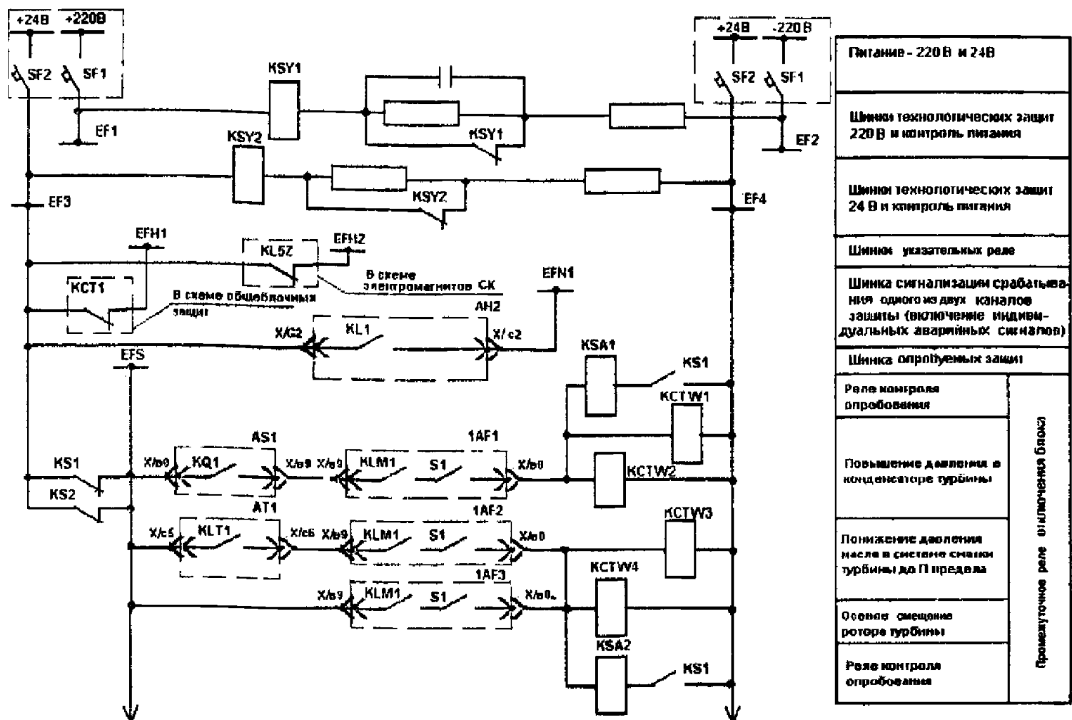
Рисунок Э.18 – Электрическая схема ТЗ турбины на УКТЗ (лист 4)
