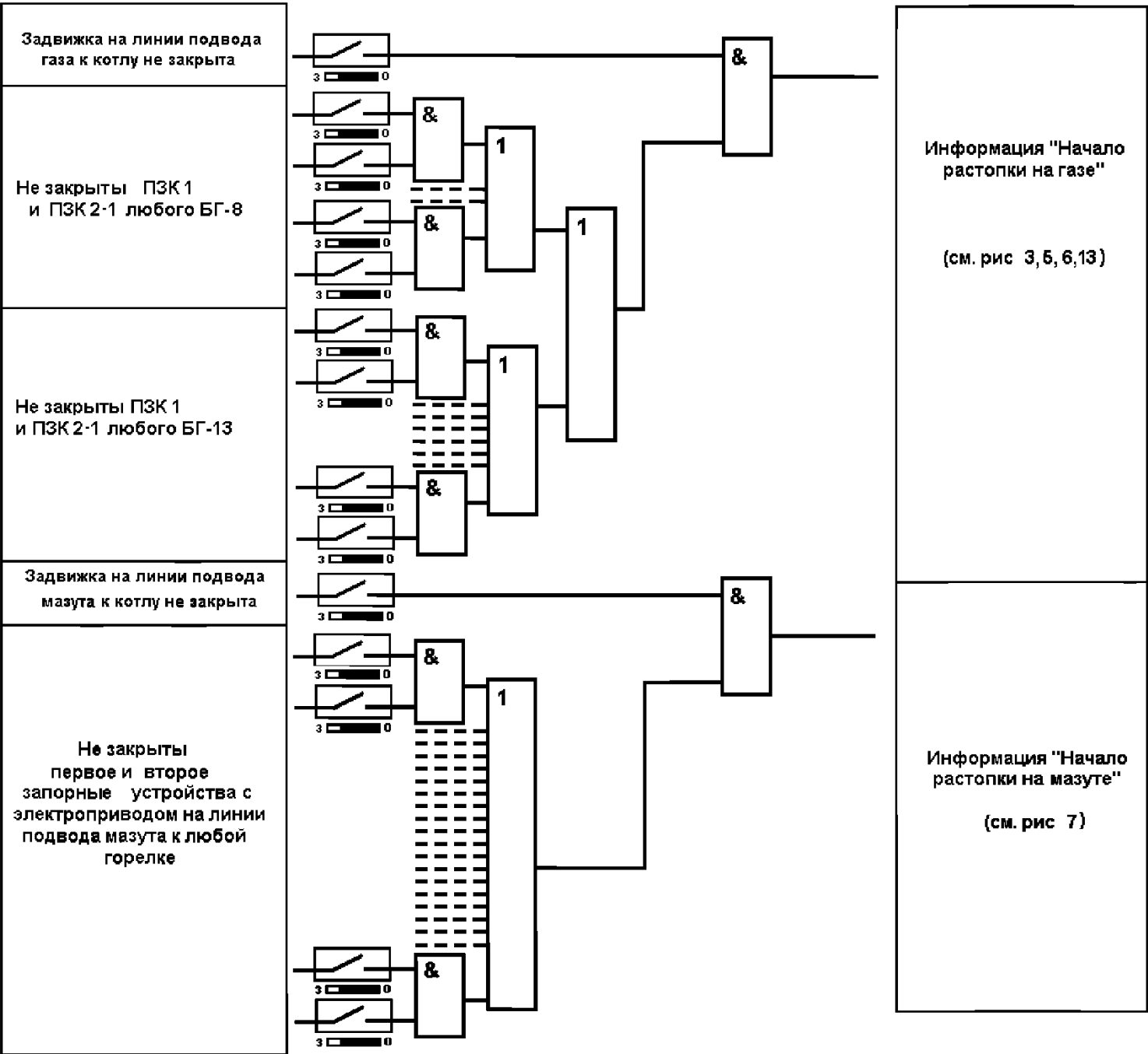
Рисунок Х.2 – Алгоритмы формирования информации «Начало растопки»
