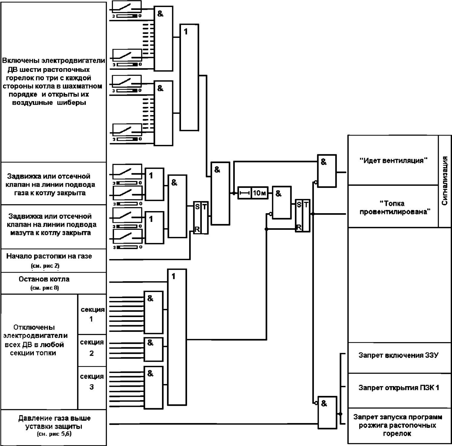
Рисунок Х.13 – Алгоритм запрета растопки котла без вентиляции топки
