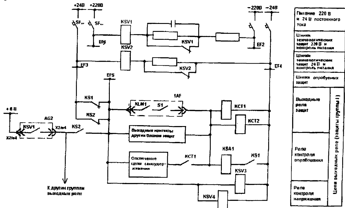
Рисунок Э.22 – Организация электрической схемы опробования ТЗ на УКТЗ (лист 1)
