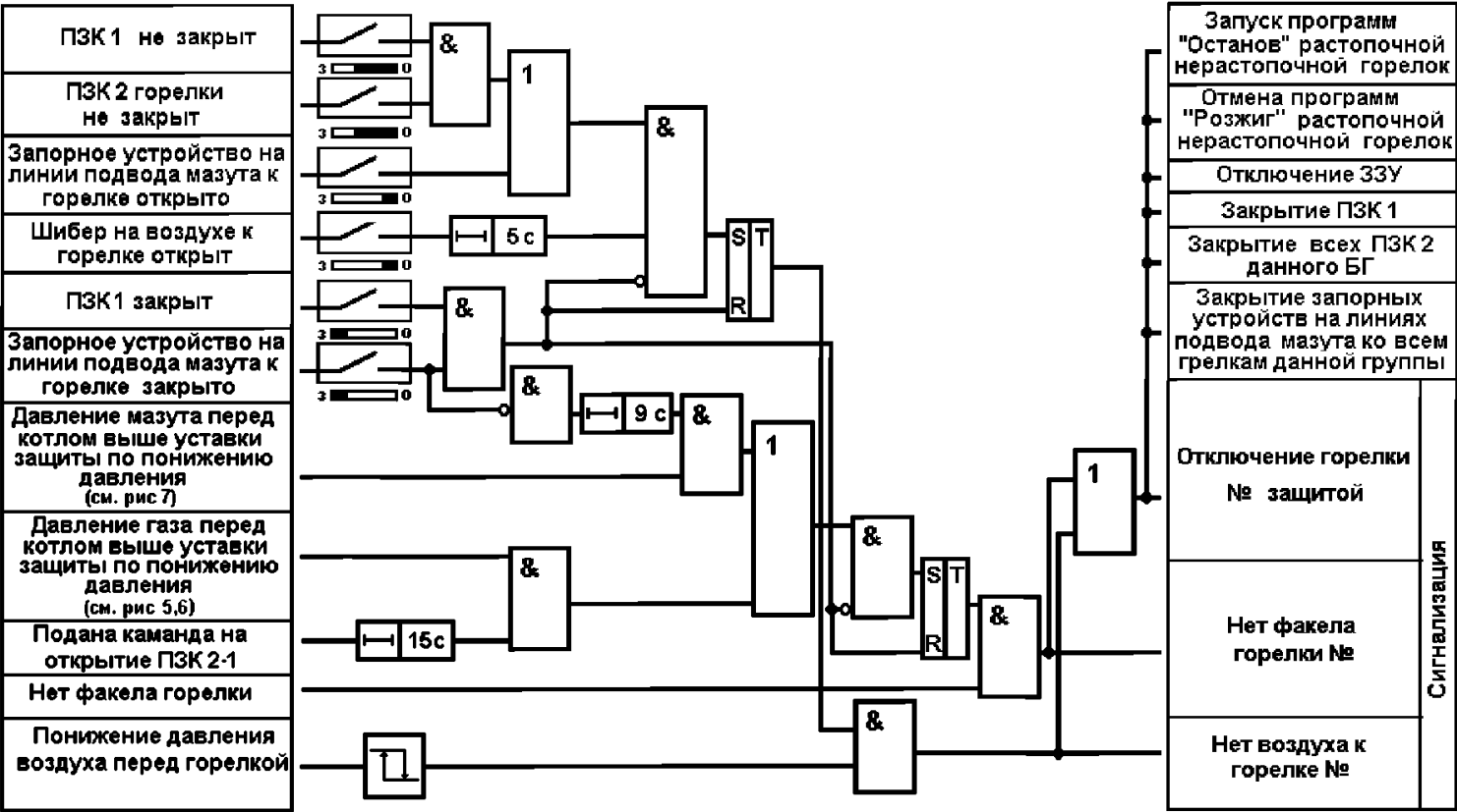
Рисунок Ш.13 – Алгоритм защит растопочной горелки котла с общими дутьевыми вентиляторами
