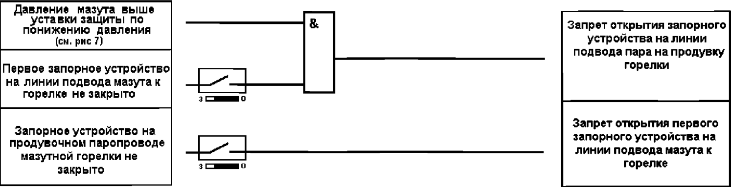
Рисунок Х.20 – Алгоритмы блокировок запорных устройств на мазуте и паре мазутной форсунки
