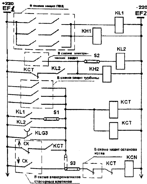
Рисунок Э.12 – Электрическая схема общекотловых защит (лист 1)
