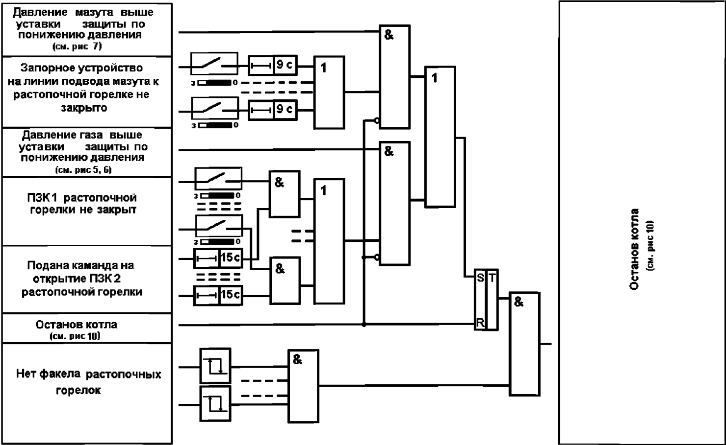
Рисунок III.4 – Алгоритм защиты «Невоспламенение первой или погасание факела всех горелок»
