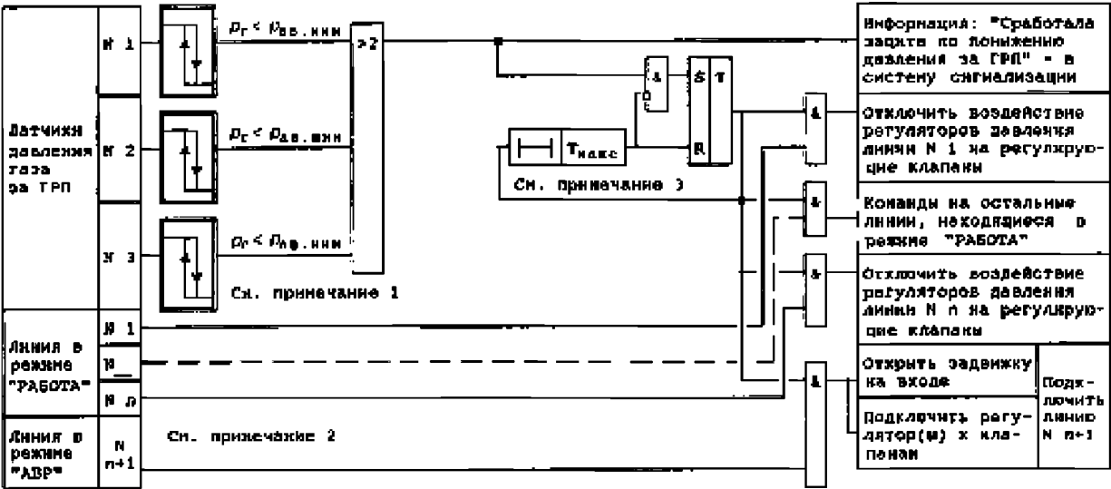
Рисунок У.3 – Структурная схема защиты по повышению давления газа за ГРП, где все элементы газопроводов до ПЗК котлов рассчитаны на давление газа до ГРП
