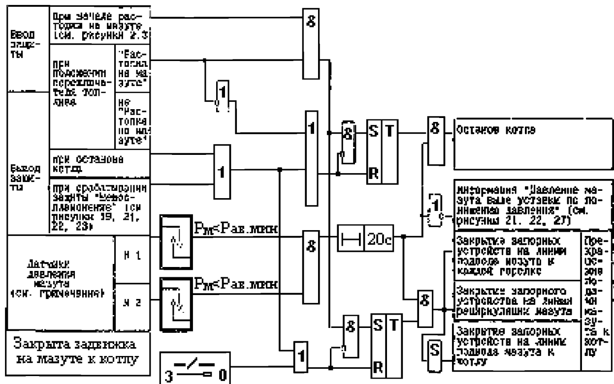
Рисунок Ф.17 - Защита по понижению давления мазута
