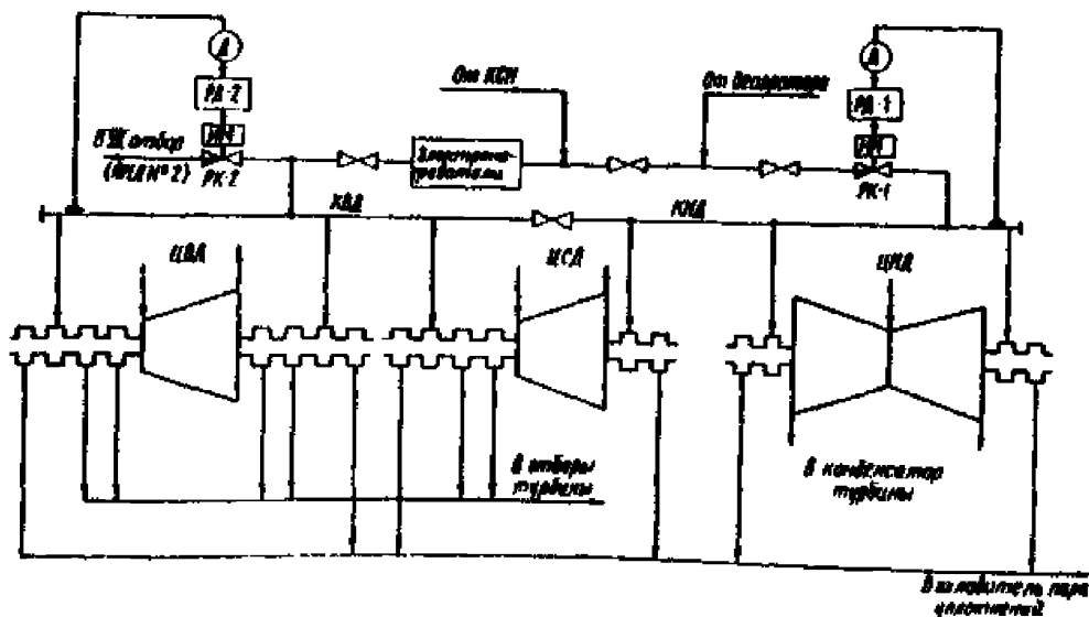
Рисунок И1.1 – Схема автоматического регулирования подачи пара на концевые уплотнения турбины К-300-240-3
