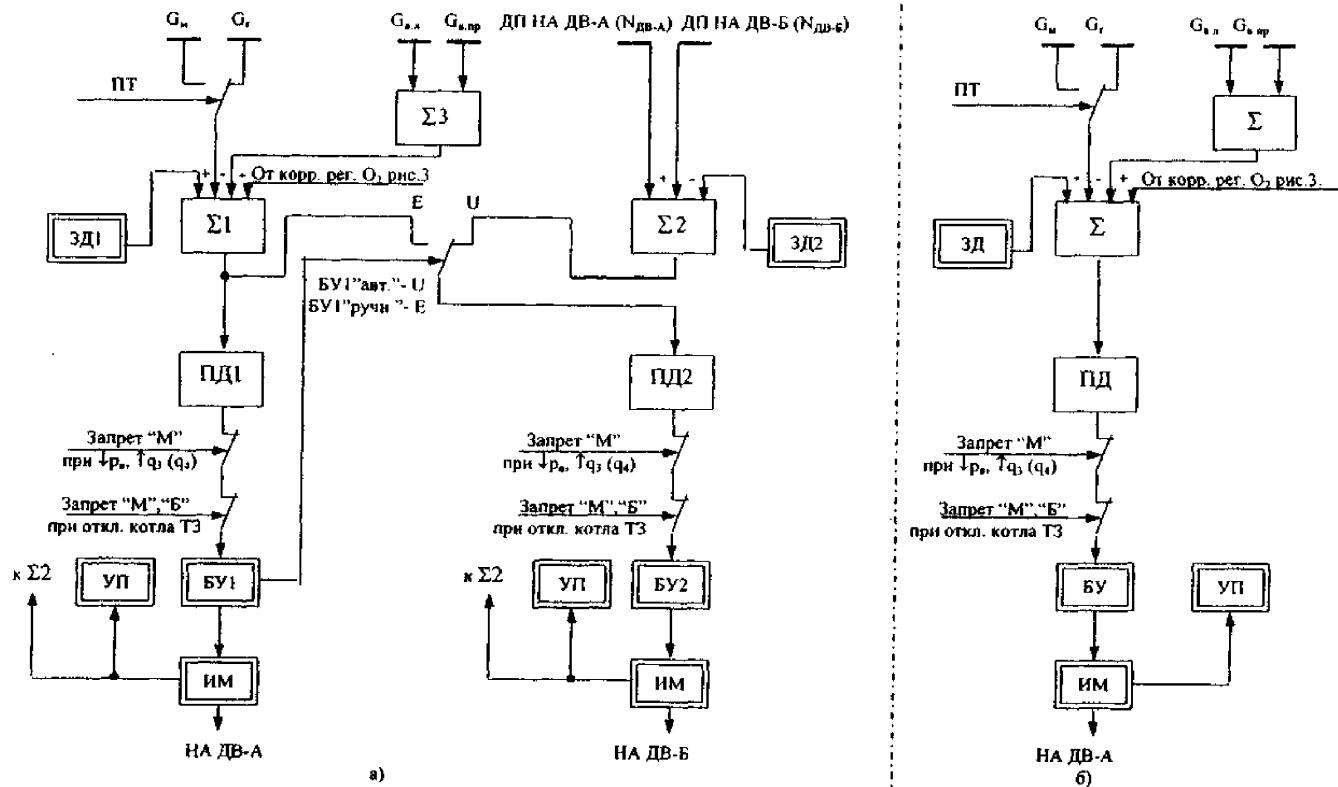
а – для котлов моноблоков; б – для котлов (корпуса) дубль-блоков Рисунок И2.2 – Структурная схема регулирования расхода общего воздуха к котлу (РОВ)
