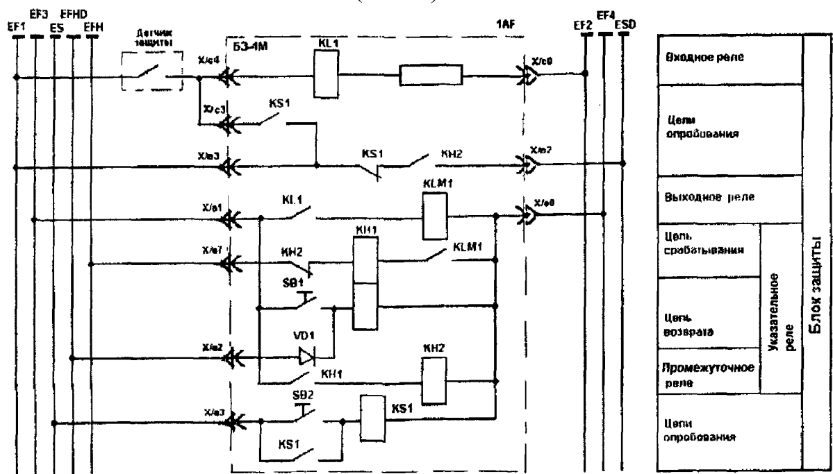
Рисунок Э.22 – Организация электрической схемы опробования ТЗ на УКТЗ (лист 2)
