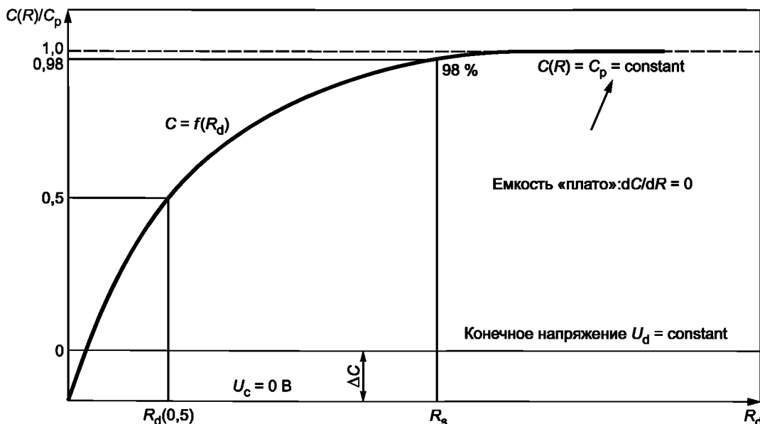
Рисунок F.1 — Нормализованная C/R диаграмма (схематично)
