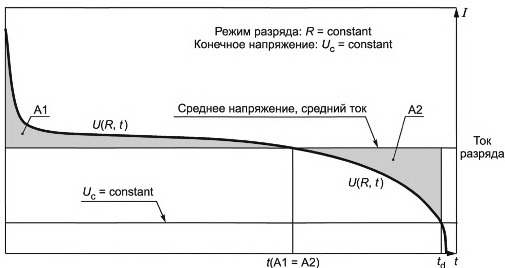
Рисунок F.2 — Стандартное напряжение разряда (схематично)
