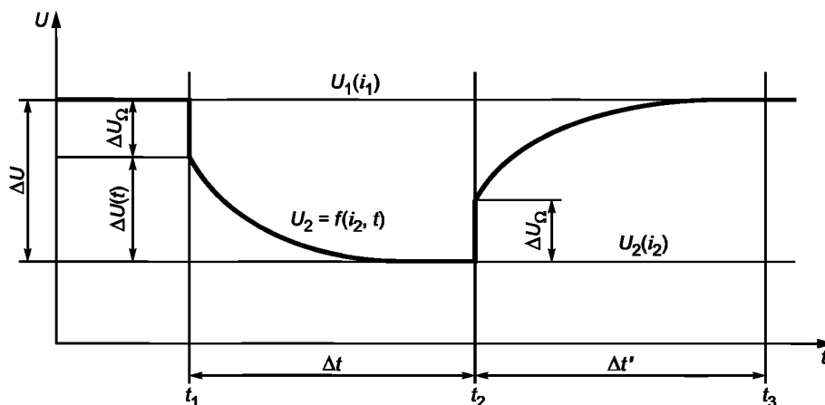
Рисунок 1 — Диаграмма изменения напряжения
