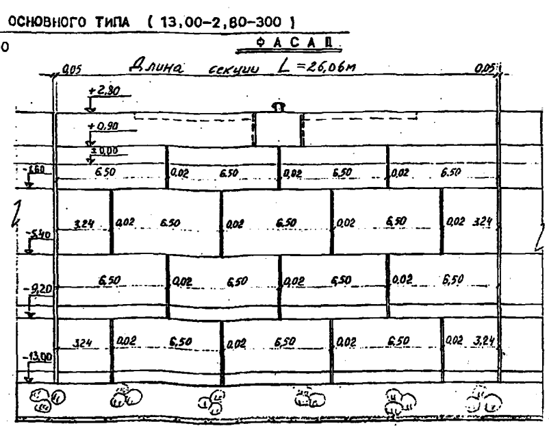
СРАВНИТЕЛЬНАЯ ТАБЛИЦА НА 100 П. М. НАБЕРЕЖНОЙ
