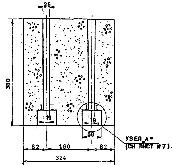
РАЗРЕЗ 2-2
