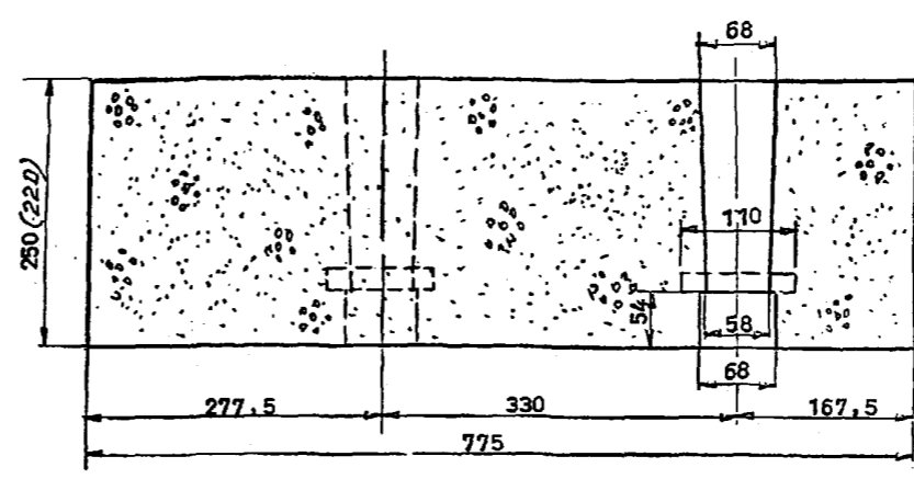
РАЗРЕЗ 1-1
