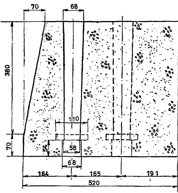
РАЗРЕЗ 1-1
