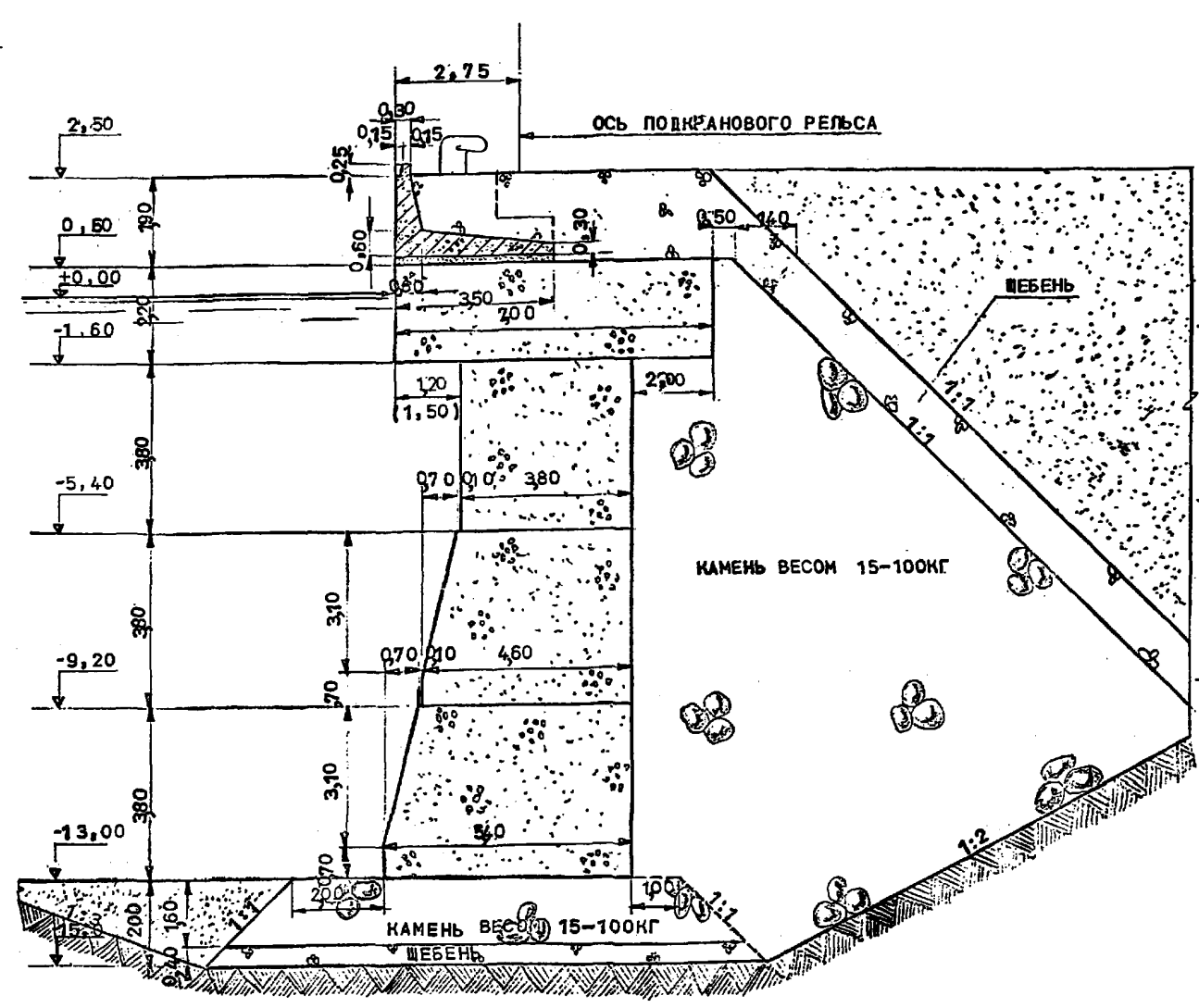
ОБЪЕМЫ РАБОТ НА 100 ПОГ. МЕТРОВ
