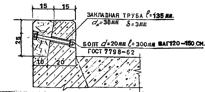
ДЕТАЛЬ КОЛЕСООТБОЙНОГО БРУСА М 1:10
