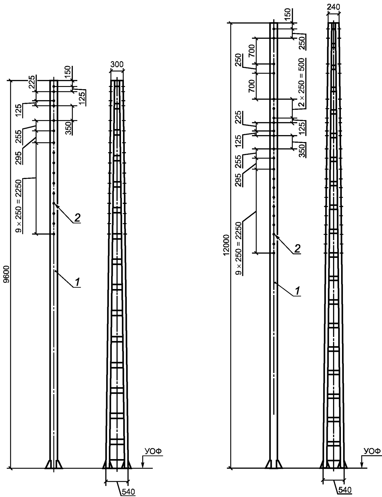
1 — стойка; 2 — отверстия для установки закладных изделий
