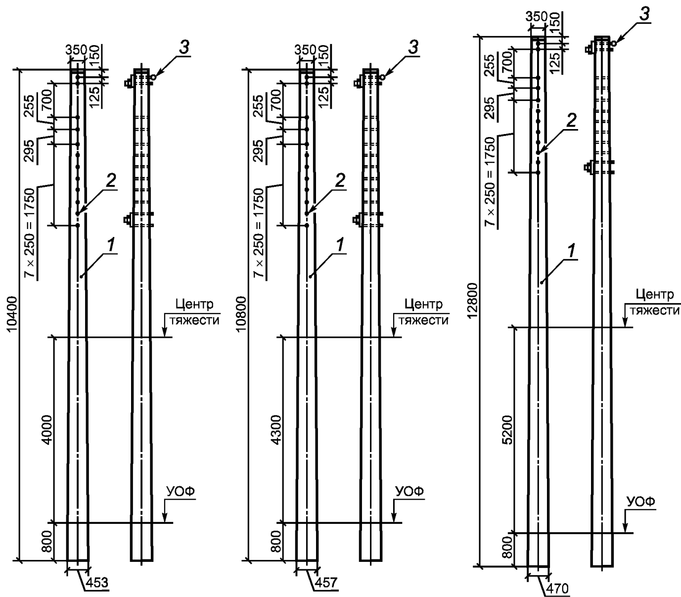
1 — стойка; 2 — отверстия для установки закладных изделий; 3 — закладные изделия
