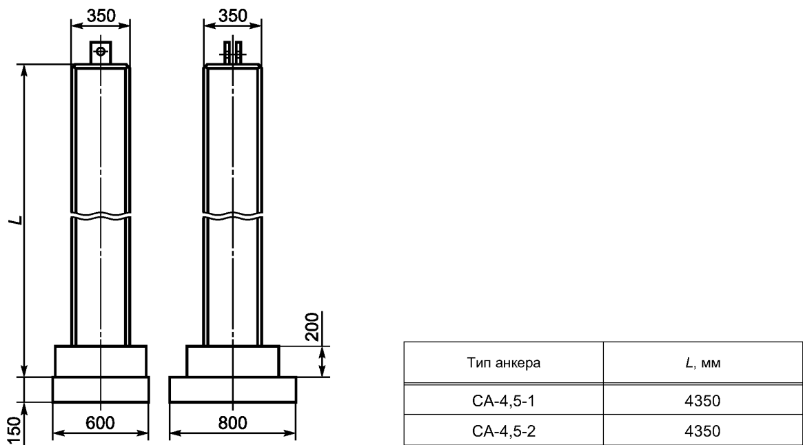
Рисунок 4 — Анкеры стоечные
