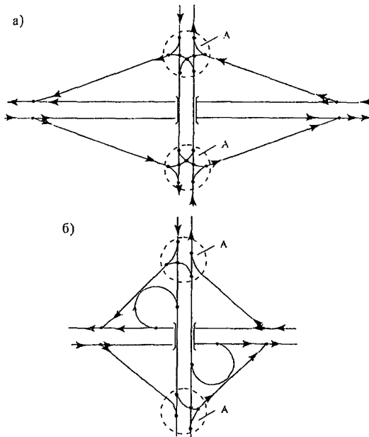
Рис. 6.1. Схема конфликтных точек на транспортных развязках неполного типа "ромб" (а), неполный "клеверный лист" (б):
