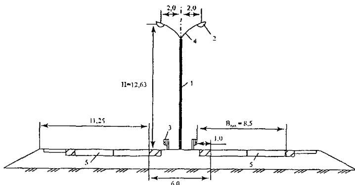
Рис. П-8.1. Поперечный профиль дороги и расположение опор светильников: 1 – опора светильника; 2 – светильник; 3 – дорожное удерживающее ограждение; 4 – крошительн; 5 – проезжая часть дороги
