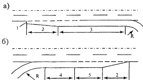
Рис. 9.3.2. Элементы полос торможения (а) и разгона (б): 1 – уступ шириной 0,5 м; 2 – участок смены полосы движения (отклонение ширины полосы); 3 – участок снижения скорости; 4 – участок ускорения; 5 – участок маневрирования
