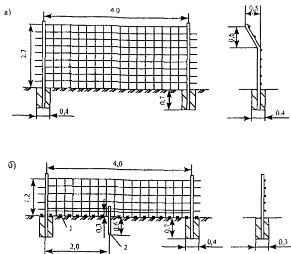
Рис. 9.10.2. Ограждения, предотвращающие выход на дорогу крупных копытных животных (а), кабанов (б): 1 – колючая проволока; 2 – дополнительный столб
