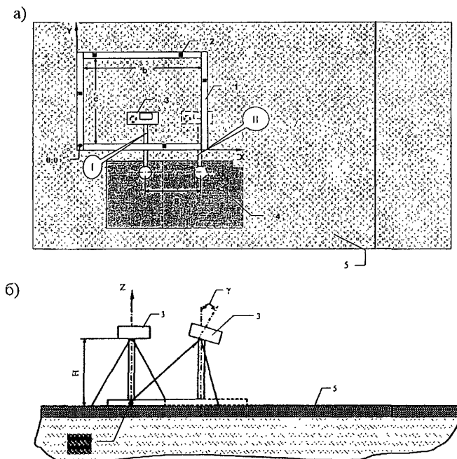
Рис. П-4.1. Схема элементов фотосъемки:
