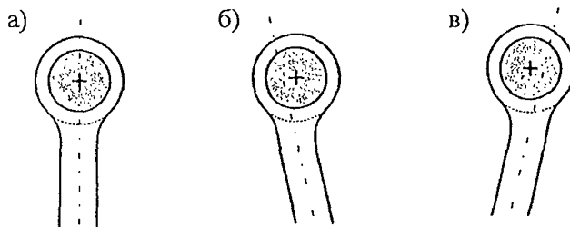
Рис. 9.2.12 Планировочные решения подходов к кольцевой проезжей части:
