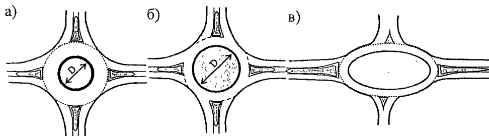
Рис. 9.2.11 Планировочные схемы кольцевых пересечений а – малый центральный островок, б – большой центральный островок, в – эллиптический центральный островок
