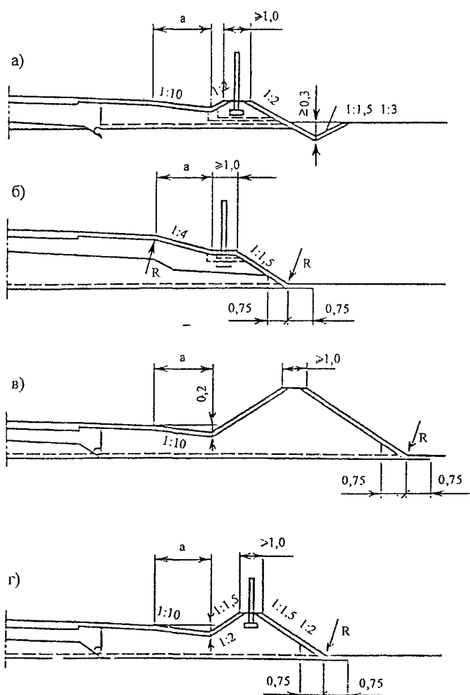
Рис. 10.5.7. Рекомендуемые поперечные профили земляного полотна для размещения на них шумозащитных сооружений:
