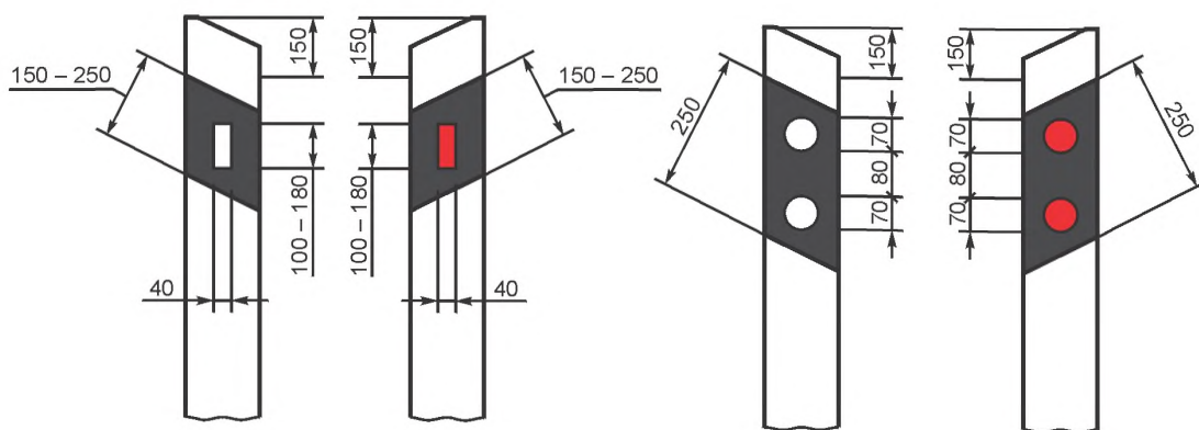
Рисунок 9 — Вертикальная разметка сигнальных столбиков, имеющих скос в верхней части корпуса
