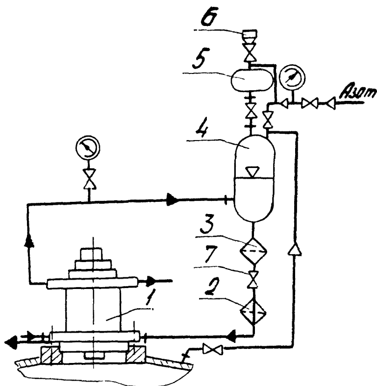
1. Схема обвязки торцовых уплотнений с естественной циркуляцией запирающей жидкости.
