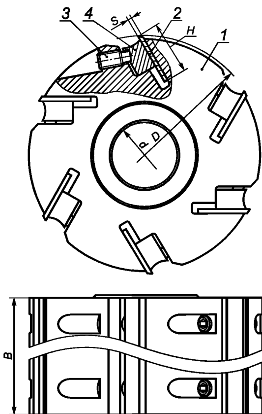
1 — корпус; 2 — нож; 3 — винт; 4 — клин
