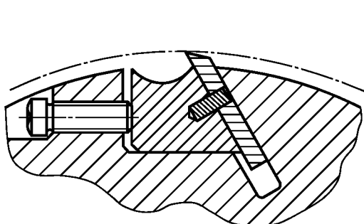
Клиновое крепление с зажимным винтом в корпусе и штифтом в клине
