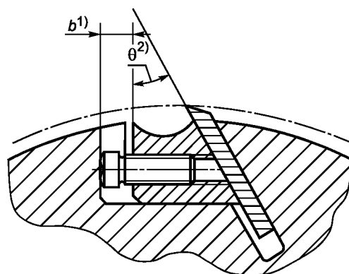
Клиновое крепление с зажимным винтом в клине 3)
