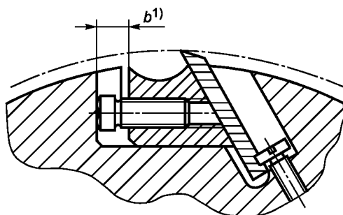
Клиновое крепление с зажимным винтом в клине и регулировочным винтом в корпусе
