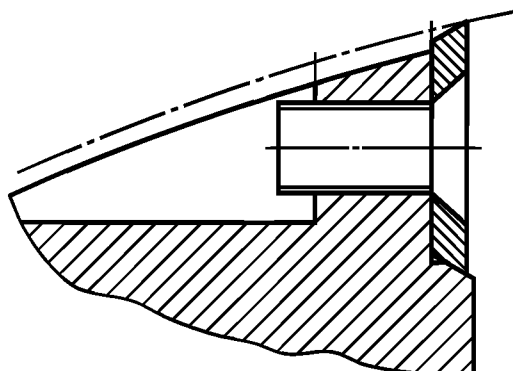
Крепление прижимным винтом со стороны передней поверхности режущей пластины
