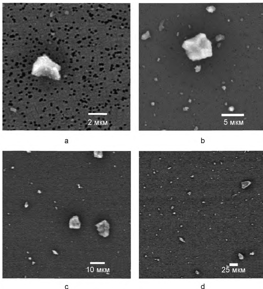
Рисунок 6 — Типичные микрографические изображения частиц ISO MTD, полученные на СЭМ при четырех увеличениях
