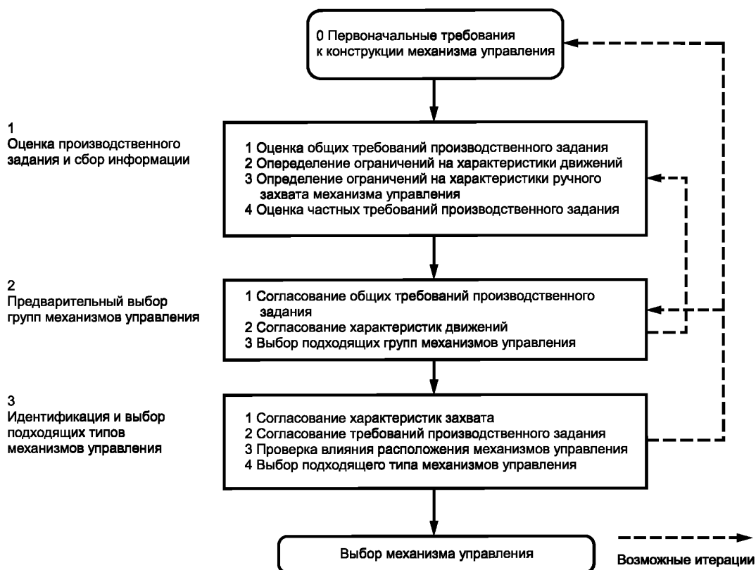
Рисунок 1 — Схема общей процедуры выбора ручного механизма управления
