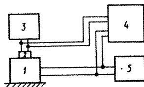
1 — вибровозбудитель; 2 — поверяемый ВИП; 3 — вольтметр; 4 — осциллограф; 5 — генератор частоты
