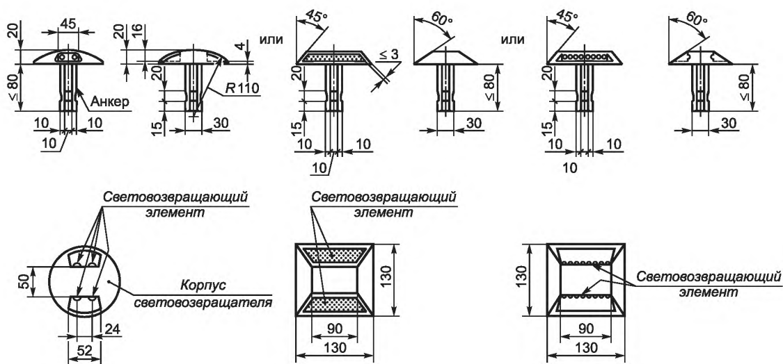
Рисунок Б.3 — Световозвращатели типа КД3
